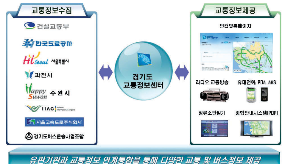
교통정보센터 정보수집 및 제공 체계도
