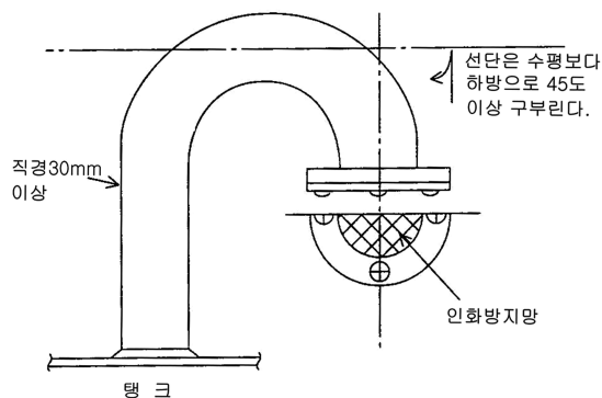
[그림 60] 밸브없는 통기관 예
