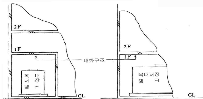
[그림 82] 상층이 있는 경우 바닥 등의 구조
