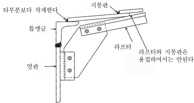
[그림 57] 이상내압방출구조의 예
