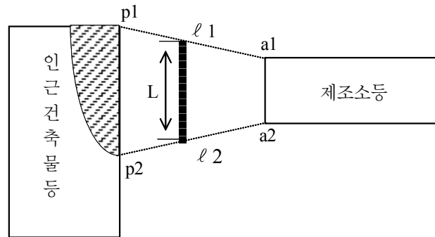
[그림 6] 방화상 유효한 담의 길이
