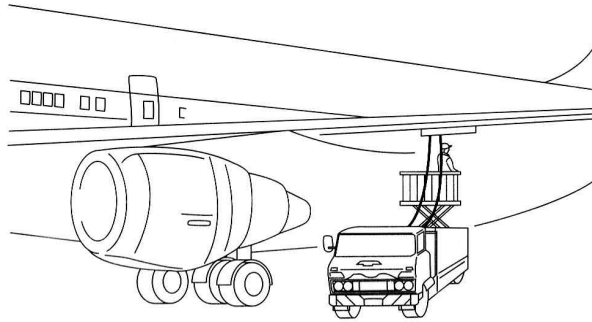
[그림 149] 주유호스차에 의한 방식 예
