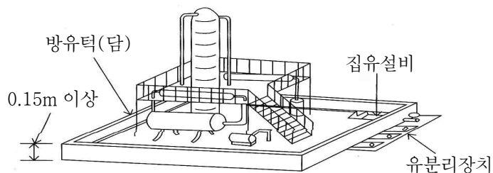
[그림 21] 옥외설비의 바닥
