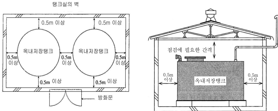
[그림 77] 탱크와 전용실간, 탱크상호간 간격
