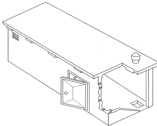
[그림 35] 지붕이 내화구조인 옥내저장소
