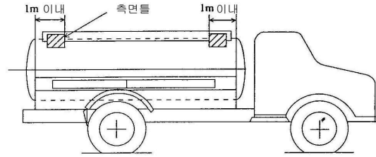
[그림 109] 측면틀 설치 위치
