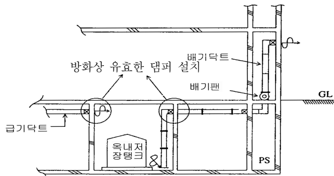
[그림 83] 탱크전용실의 환기설비 예
