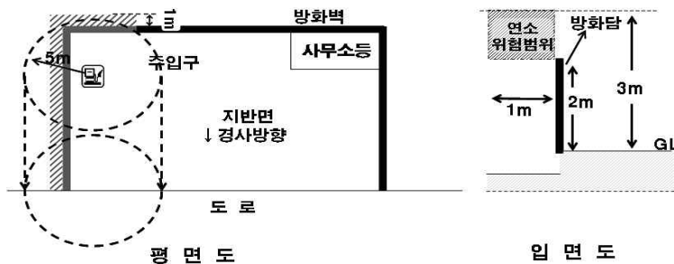
[그림 146] 제2종 연소범위 예
