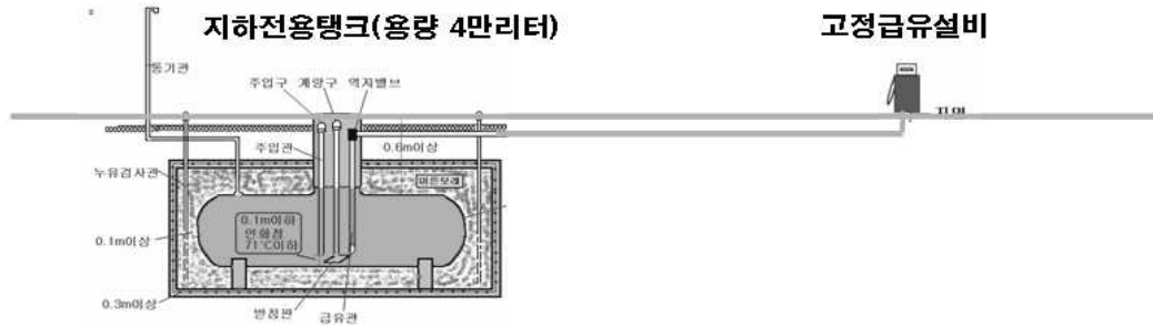
[그림 181] 옮겨 담은 일반취급소의 구성
