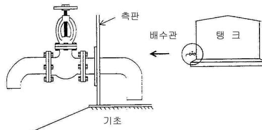
[그림 69] 배수관의 설치 예
