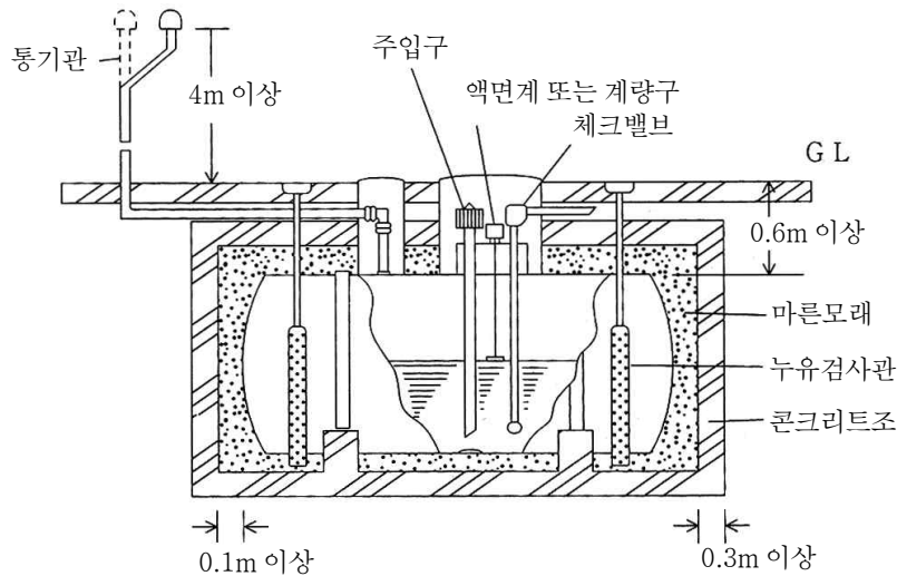
[그림 86] 탱크전용실에 설치된 지하저장탱크
