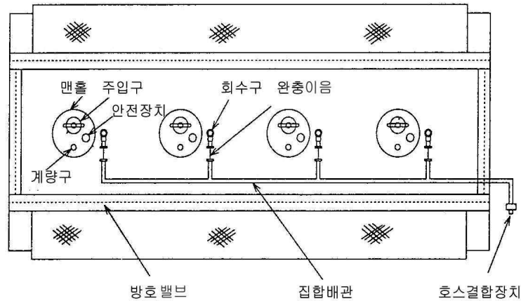
[그림 115] 집합배관을 설치 회수호스를 연결하는 방식
