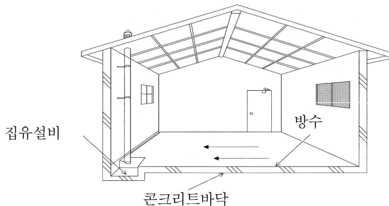
[그림 36] 옥내저장소의 바닥
