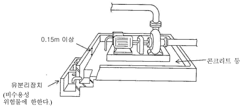
[그림 67] 펌프실 외에 설치된 펌프
