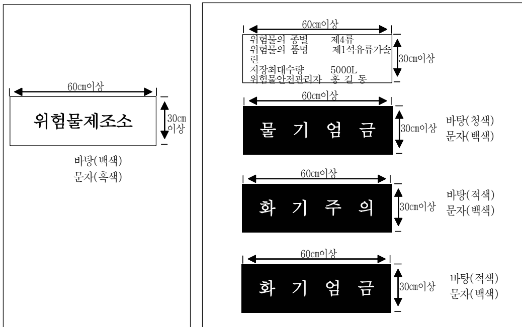
[그림 10] 표지 및 게시판
