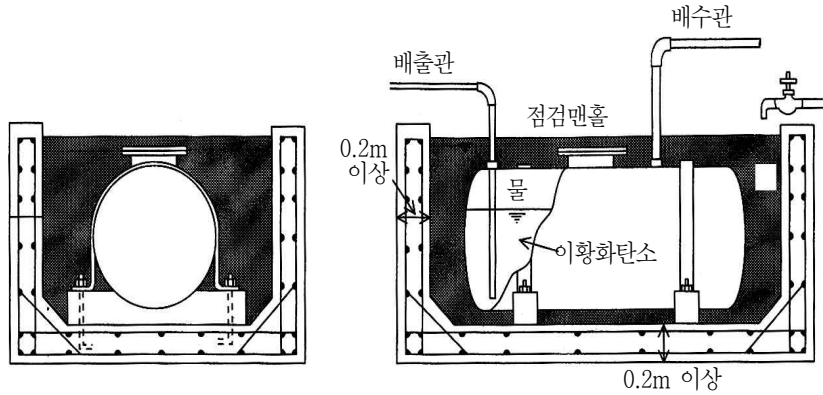
[그림 75] 이황화탄소의 저장탱크
