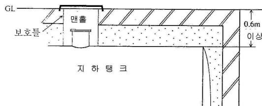
[그림 89] 탱크의 매설깊이
