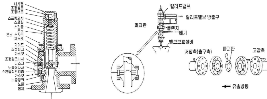
[그림 25] 안전밸브 및 파괴판
