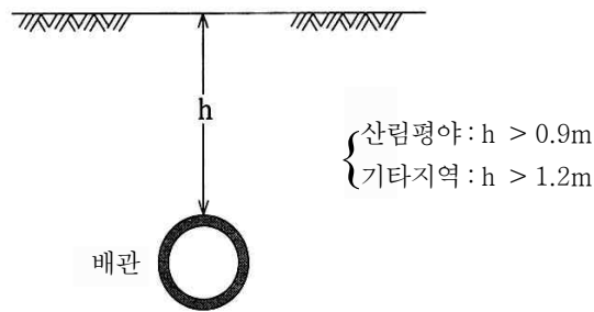
[그림 160] 지해배관의 지표면으로부터의 거리
