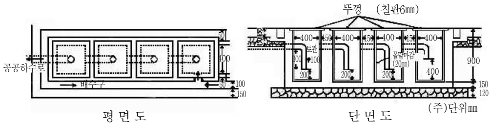
[그림 22] 유분리장치
