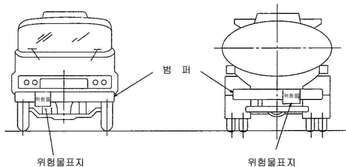
[그림 116] 표지판의 설치
