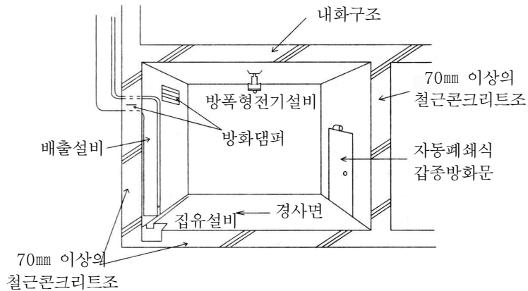
[그림 176] 분무도장작업등의 일반취급소의 건축물 구조
