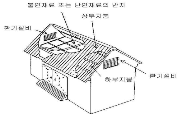
[그림 38] 온도 상승방지조치 예
