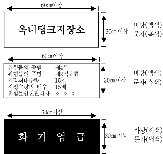
[그림 79] 표지 및 게시판의 예
