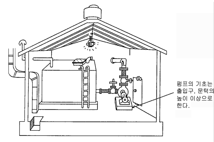
[그림 81] 펌프가 탱크전용실 내에 설치된 경우
