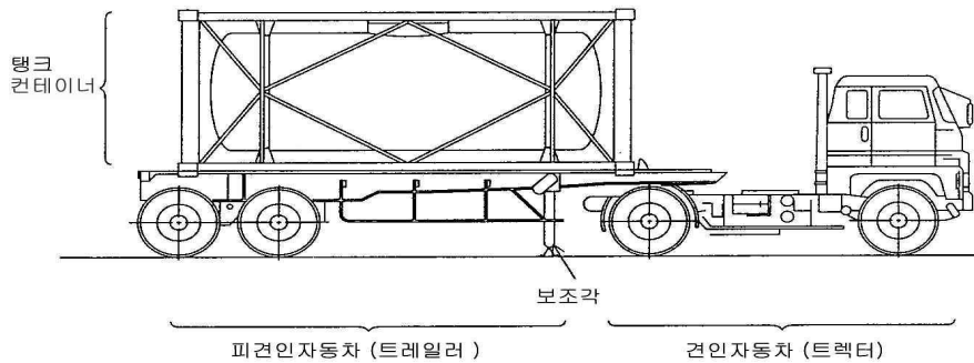
[그림 117] 컨테이너식 이동탱크저장소의 예
