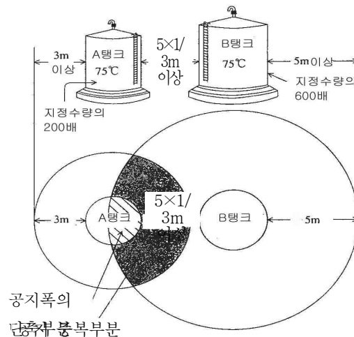
[그림 54] 공지단축되는 예
