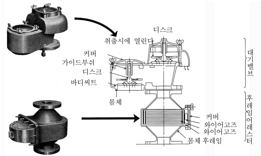
[그림 63] 대기밸브 부착 통기관
