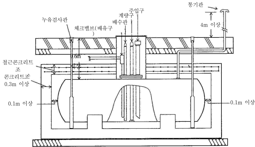
[그림 88] 전용실의 구조
