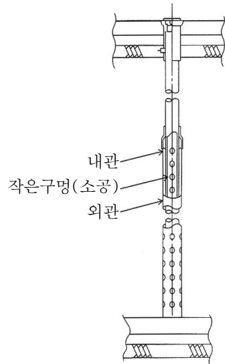
[그림 94] 누유검사관
