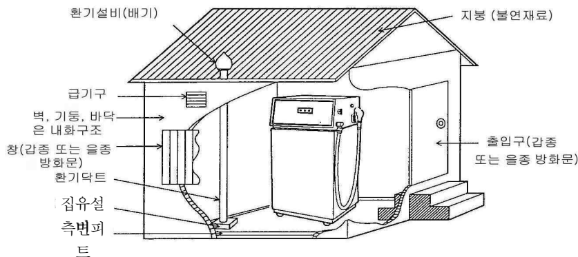
[그림 101] 옥내에 설치하는 간이탱크저장소
