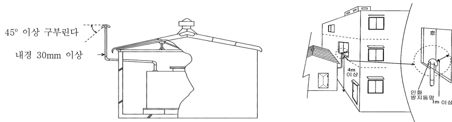
[그림 80] 통기관의 설치 예
