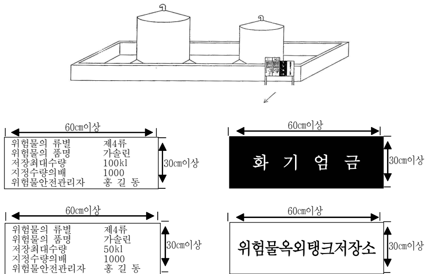
[그림 56] 표지 및 게시판의 예
