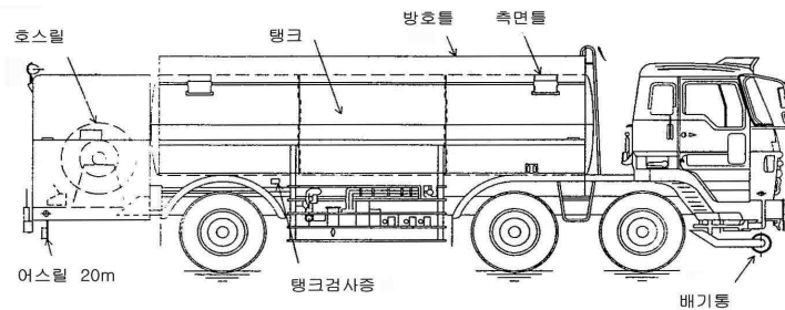
[그림 120] 주유탱크차 예
