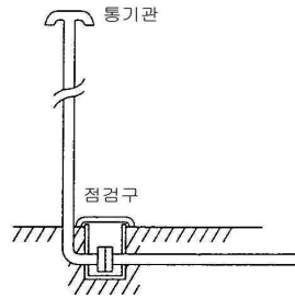
[그림 92] 통기관의 점검구
