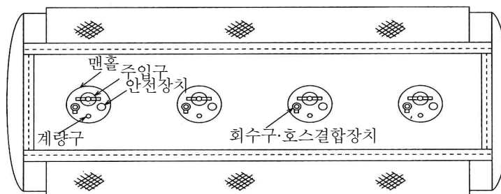
[그림 114] 회수호스를 회수구에 직접 연결하는 방식 예
