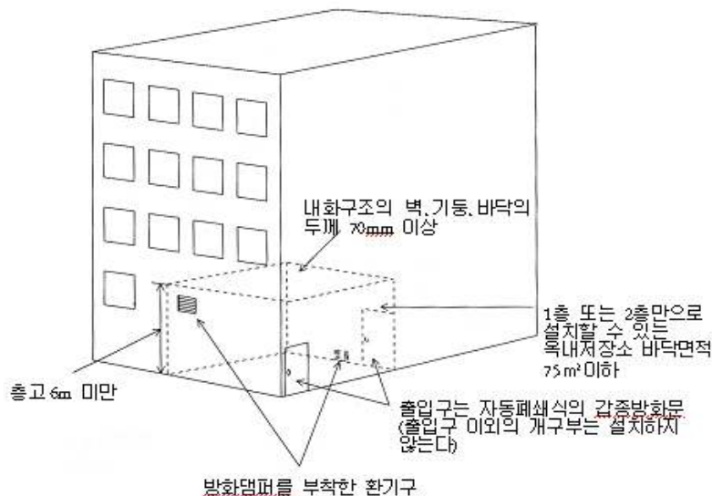
[그림 40] 복합용도 건축물의 옥내저장소
