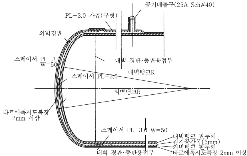
[그림 97] 강제이중벽탱크의 구조
