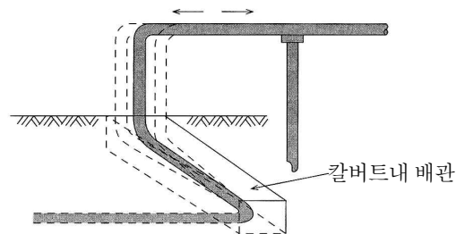
[그림 158] 굽은 관에 의한 신축흡수 조치
