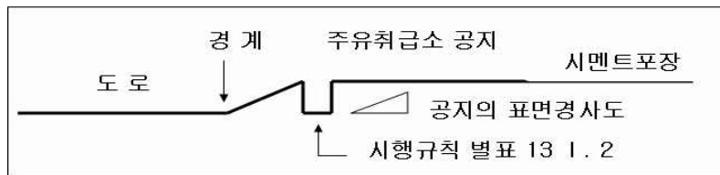
[그림 130] 주유설비의 바닥
