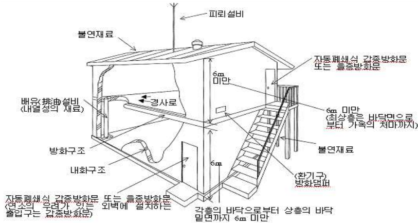
[그림 39] 다층 건물의 옥내저장소
