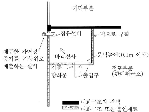
[그림 156] 배합실의 설치 예
