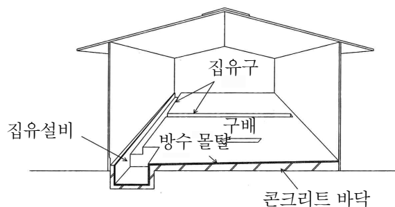
[그림 15] 액체위험물을 취급하는 건축물의 바닥
