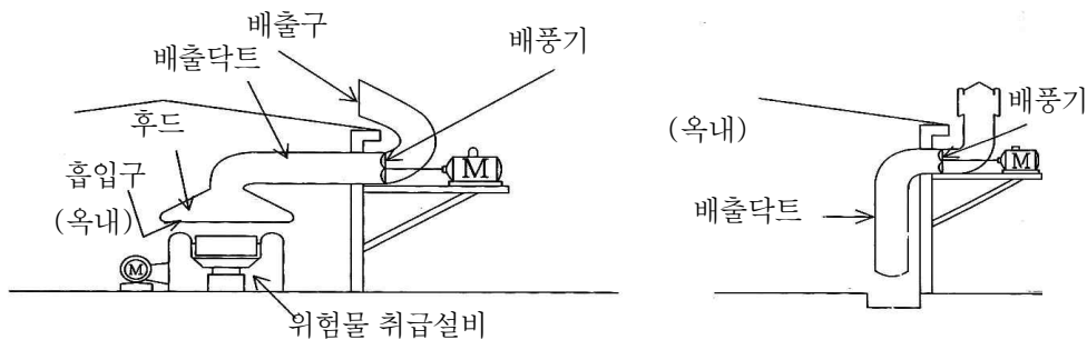
[그림 19] 배출설비의 구성
