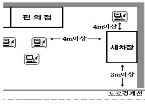
[그림 140] 세차장의 설치 예
