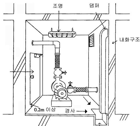
[그림 84] 펌프를 탱크전용실 외의 장소에 설치 예
