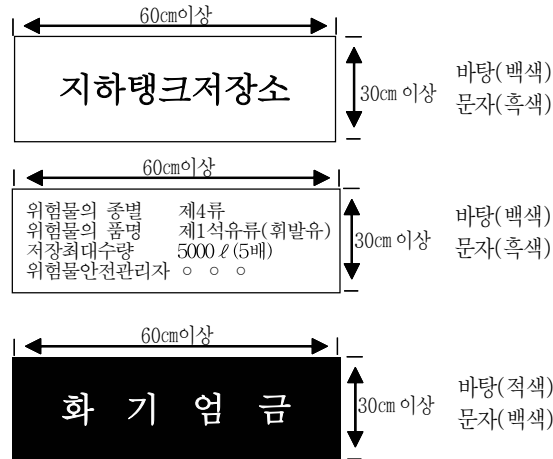
[그림 90] 표지 및 게시판의 예
