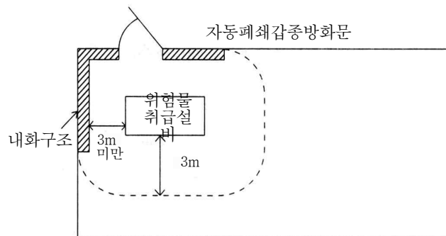
[그림 177] 공지 예
