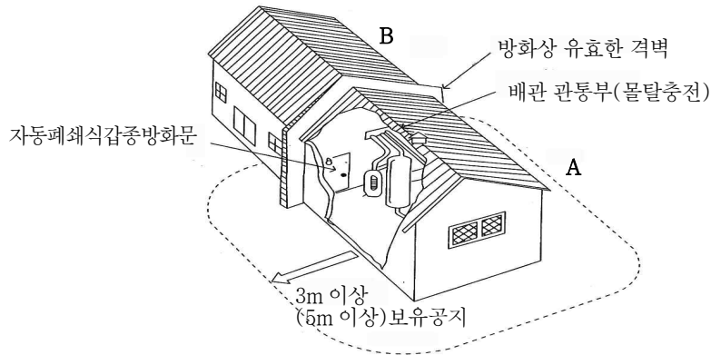
[그림 9] 보유공지의 적용 예외
