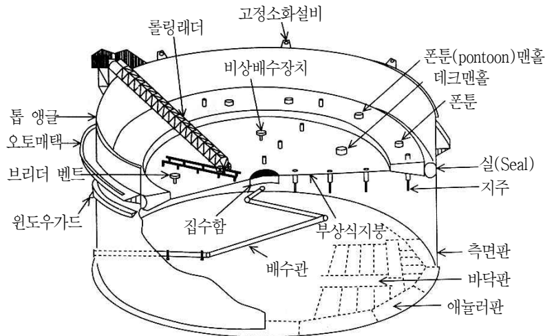
[그림 72] 부상지붕 옥외저장탱크
