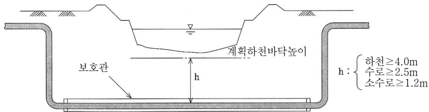
[그림 169] 하천 횡단시 하천 밑에 매설 예
