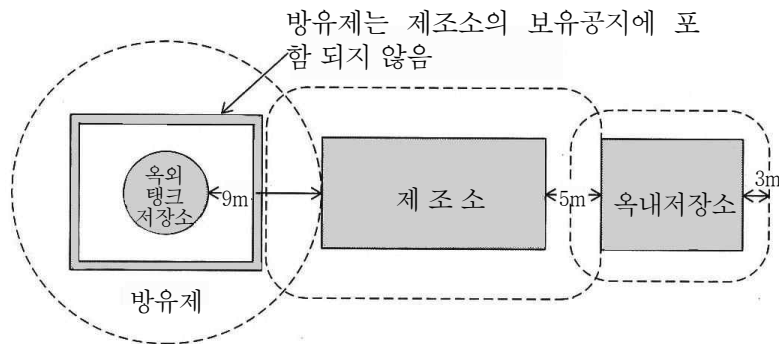
[그림 8] 보유공지의 중복
