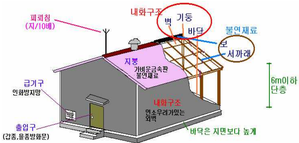
[그림 33] 옥내저장소의 구조
