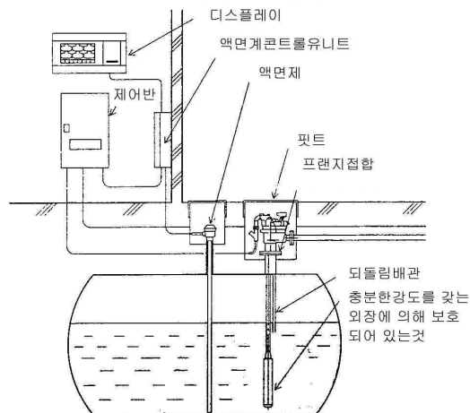
[그림 93] 액중펌프의 설치 예
