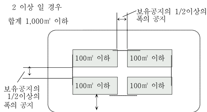
[그림 124] 면적제한 및 간격 예
