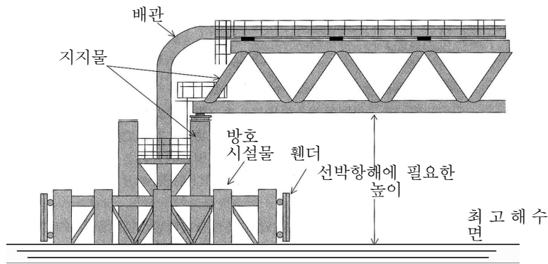
[그림 166] 배관의 해상설치 예
