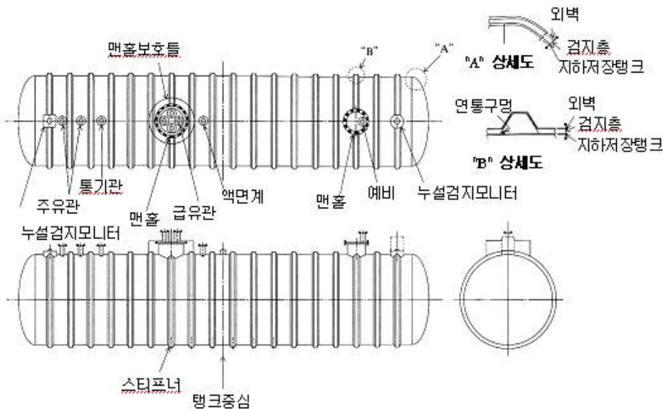
[그림 99] 강화플라스틱제 이중벽탱크의 구조
