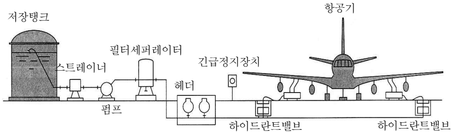
[그림 148] 주유배관 및 호스기기에 의한 방식 예
