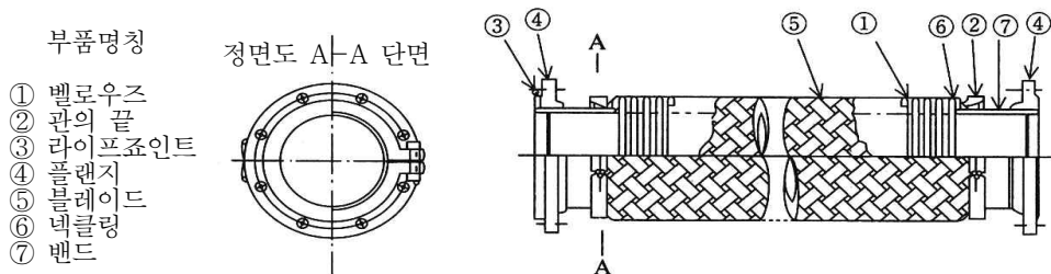
[그림 71] 플렉시블미터호스
