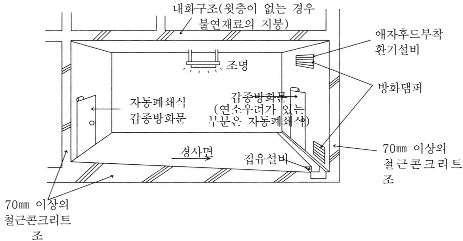
[그림 179] 지정수량 30배 미만의 열처리작업등의 일반취급소 예
