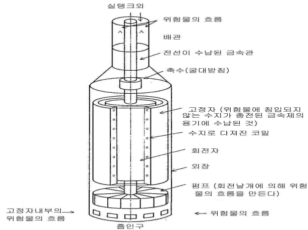
[그림 92] 액중펌프 예
