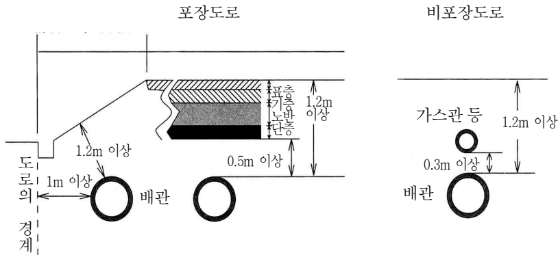
[그림 162] 시가지 외의 도로 노면밑에 매설
