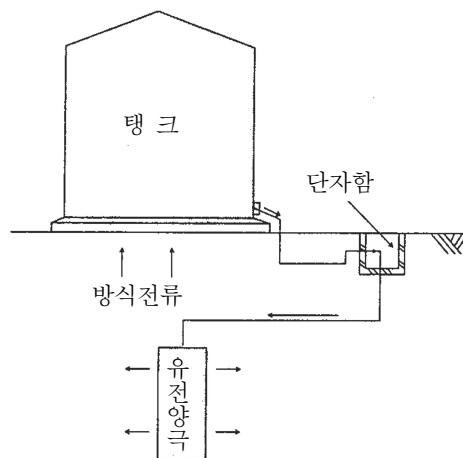
[그림 59] 전기방식의 예
