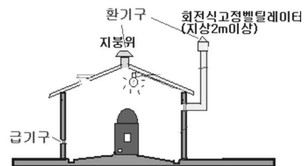
[그림 18] 환기설비
