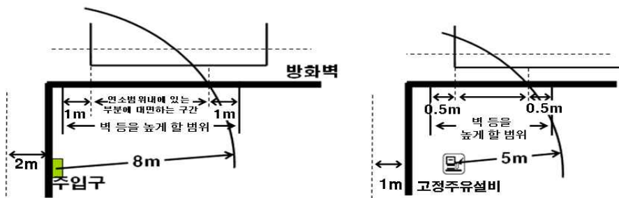
[그림 147] 벽을 높게 해야 할 범위
