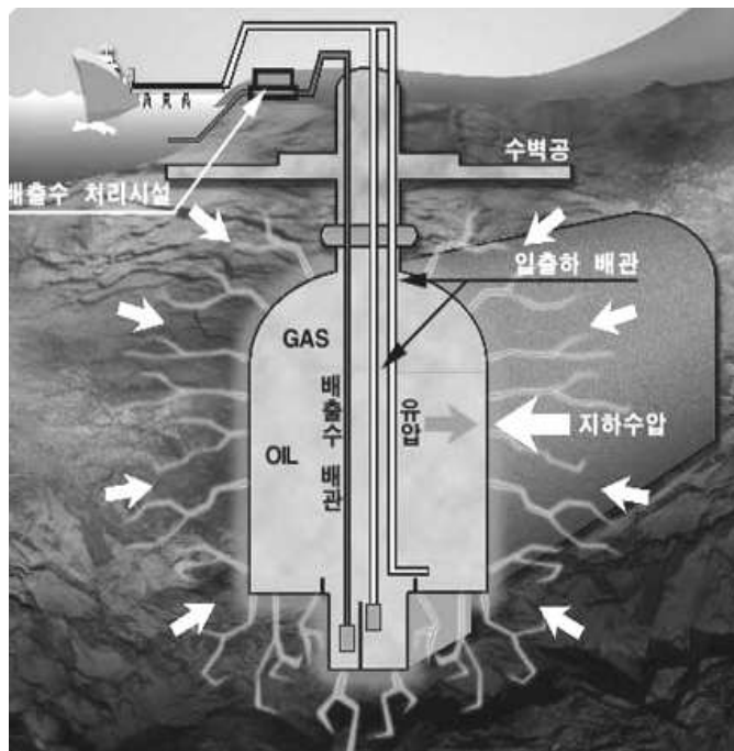
[그림 128] 암반탱크저장소 저장원리
