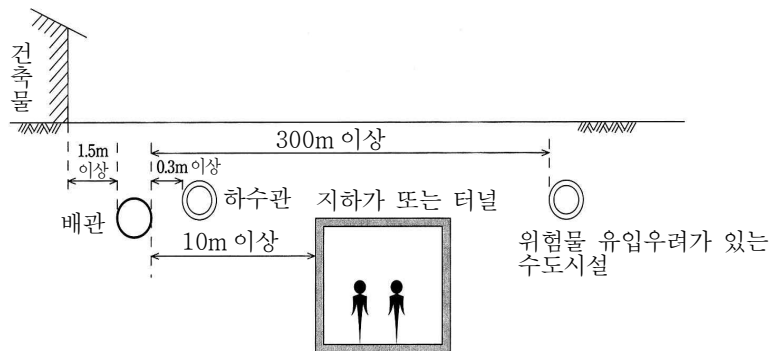
[그림 159] 배관과 건축물등과의 수평거리
