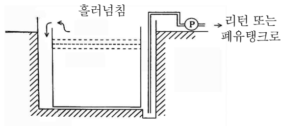
[그림 23] 되돌림관 설치 예
