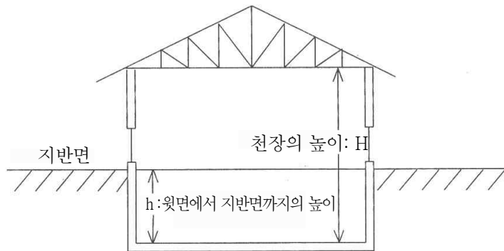
[그림 11] 지하층에 해당하는 경우( h \geq H/2 )
