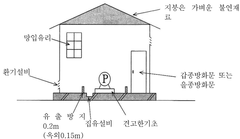
[그림 173] 펌프실의 구조 예
