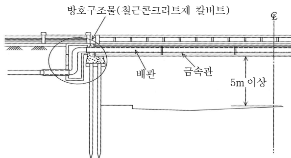
[그림 168] 도로 상공 횡단 설치 예
