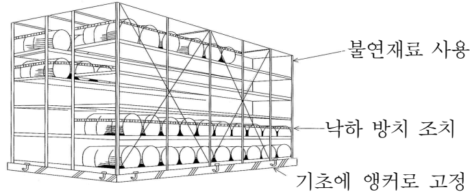
[그림 37] 옥내저장소의 선반 구조
