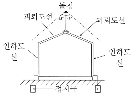
[그림 26] 피뢰설비 설치 예
