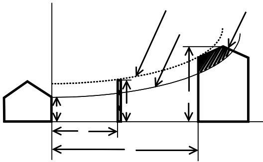
[그림 5] 방화상 유효한 담의 높이 산정
