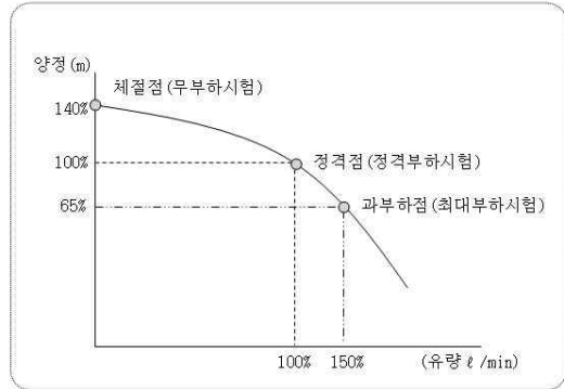
[소방펌프의 특성곡선]
