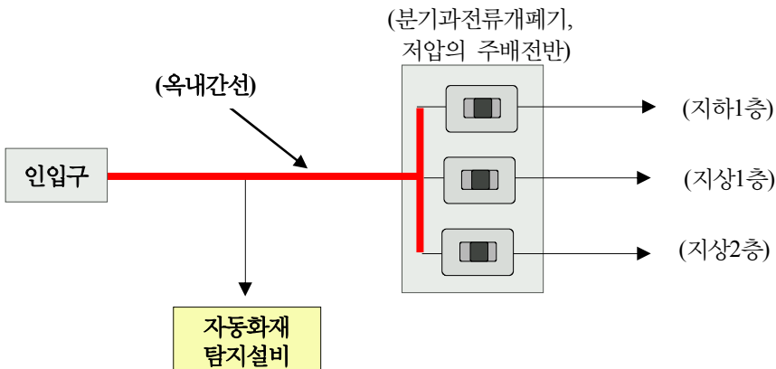
[그림 5-4] 자동화재탐지설비 상용전원의 분기
