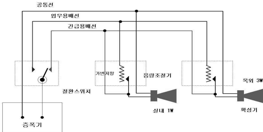
[그림 2-81] 3선식 배선의 결선
