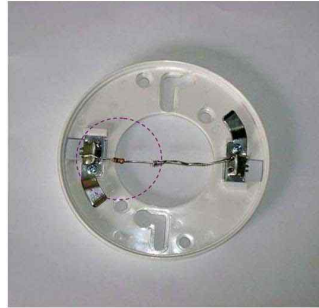
[그림 2-52] 종단저항 설치(발신기세트함 및 종단감지기)
