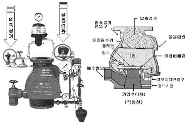
[그림 4-10] 건식밸브 구조
