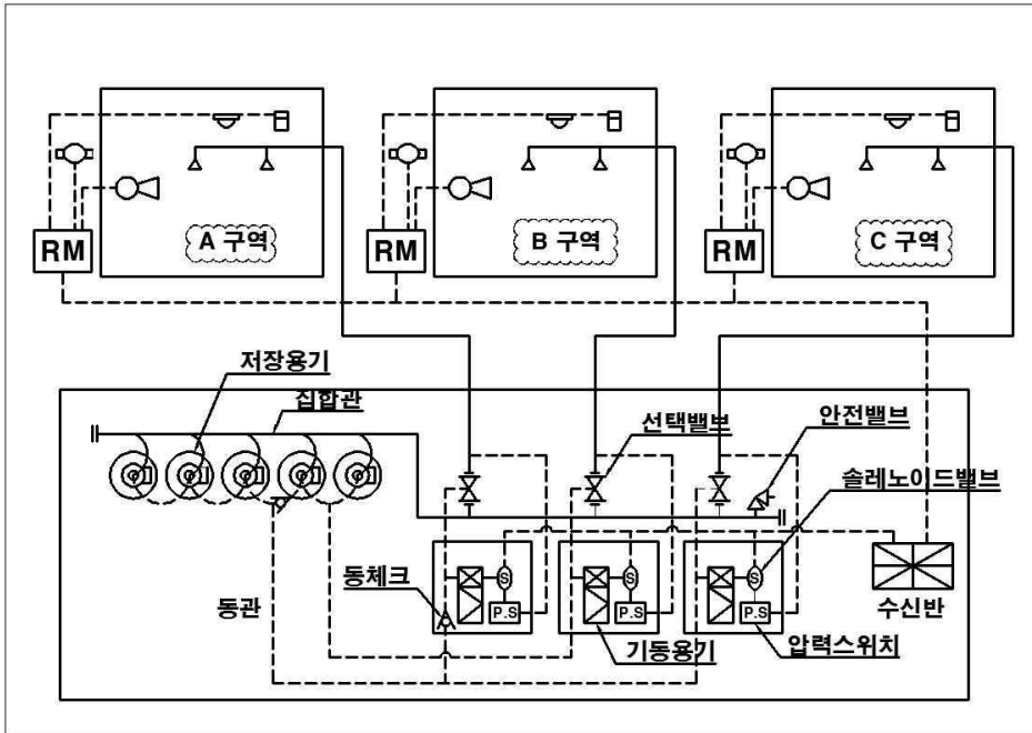
[그림 6-1] 이산화탄소설비 계통도
