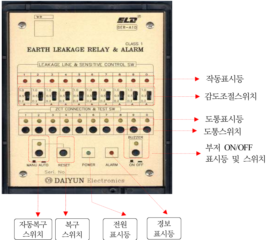
[그림 2-71] 누전경보기의 표시등 및 스위치
