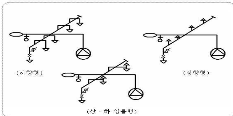
[그림 4-17] 헤드설치방법
