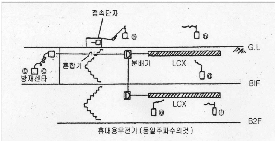
[그림 3-22] 무선통신보조설비의 사용
