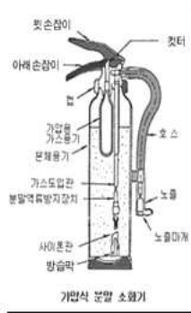
[그림 2-8] 가압식 분말소화기 점검
