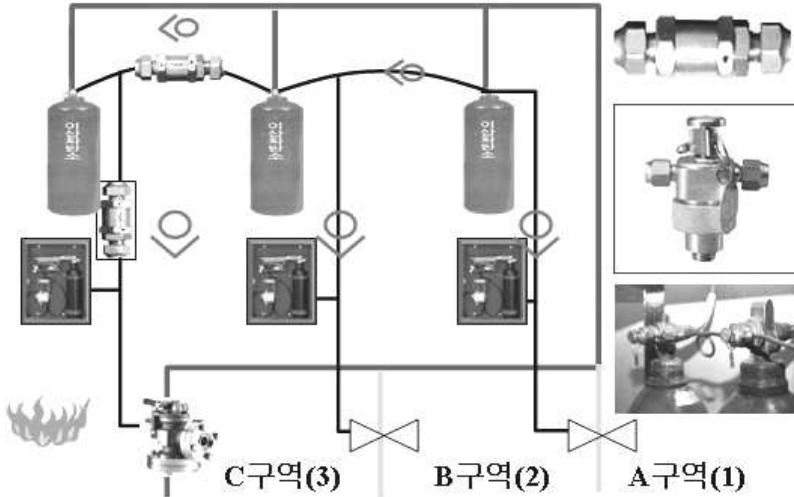
[그림 6-3] 방호구역과 선택밸브
