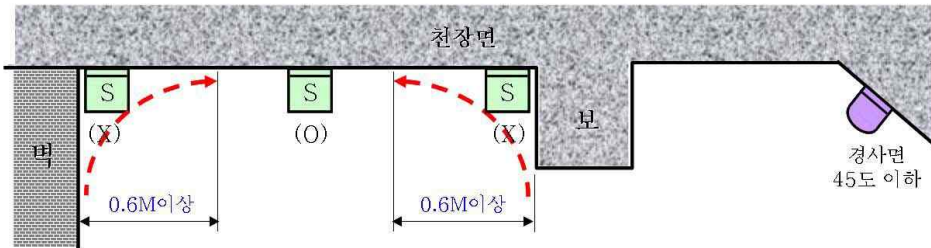
[그림 2-32] 벽 및 보로부터의 감지기의 설치위치
