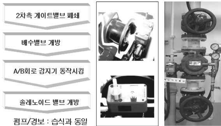
[그림 4-26] 준비작동식 점검
