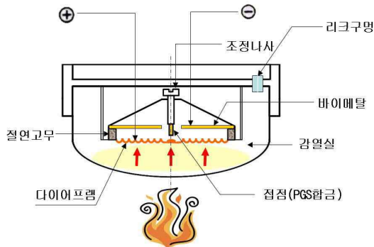
[그림 2-18] 보상식감지기 구조
