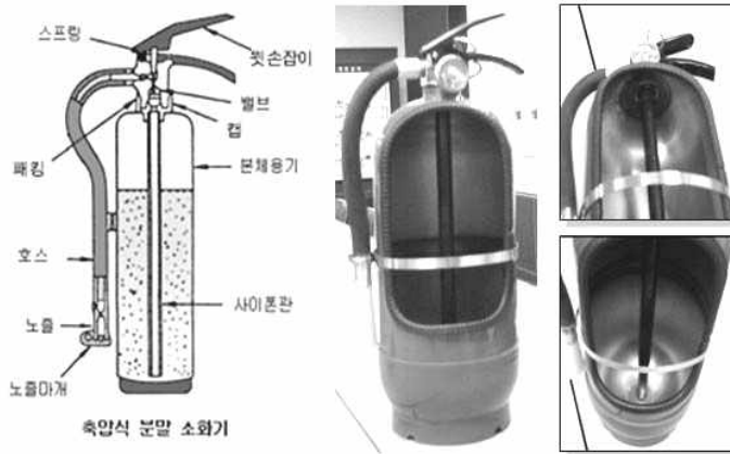
[그림 2-2] 축압식 분말소화기 구조
