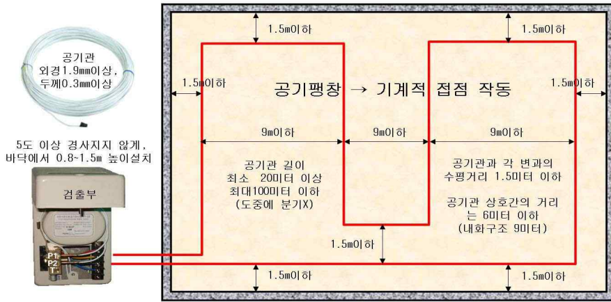
[그림 2-34] 공기관식 감지기의 설치기준
