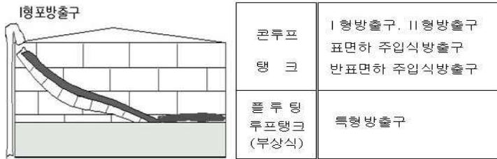
[그림 5-14] I형 방출구
