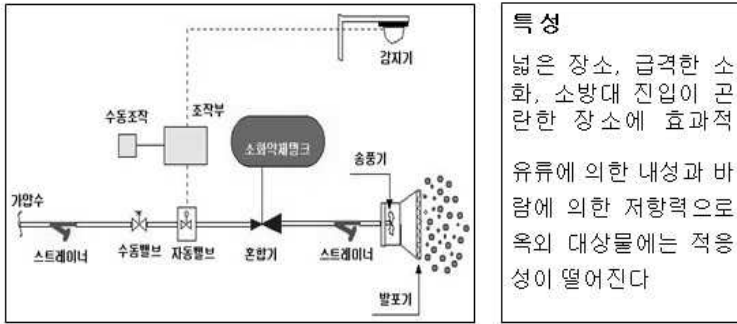
[그림 5-19] 고발포형 고정포 방출구
