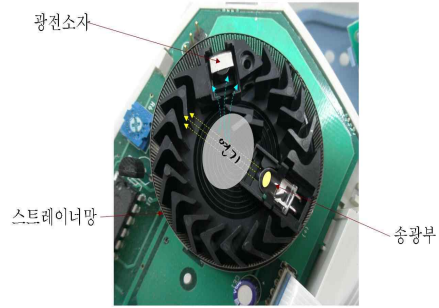
[그림 2-23] 산란광식의 내부
