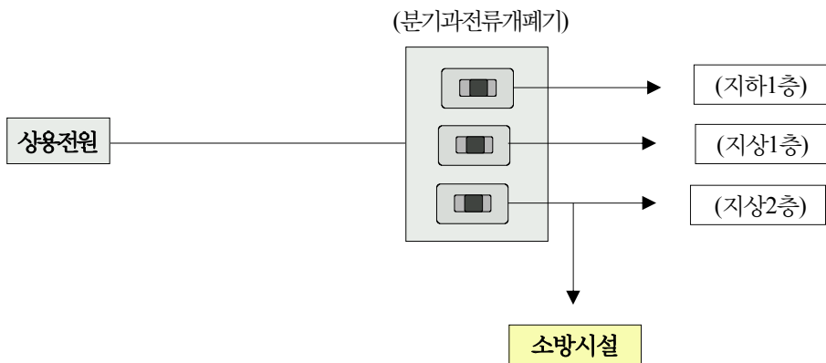
[그림 5-2] 소방시설 상용전원의 분기(×)
