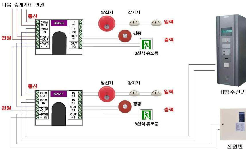
[그림 2-56] 분산형 중계기 계통배선
