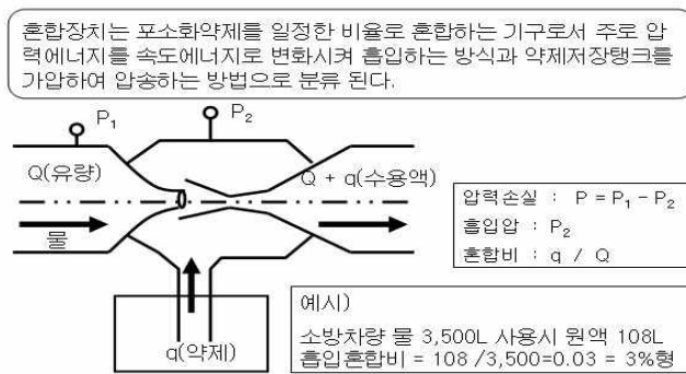
[그림 5-5] 포소화약제 혼합장치
