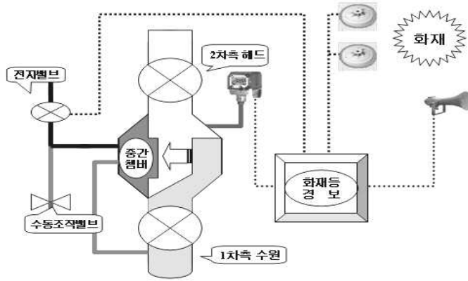
[그림 4-6] 준비작동식밸브 교차회로방식
