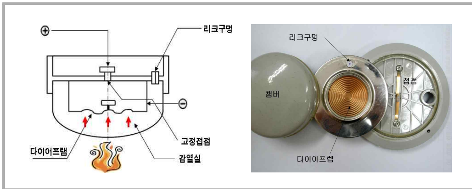
[그림 2-4] 차동식스포츠형 감지기 구조
