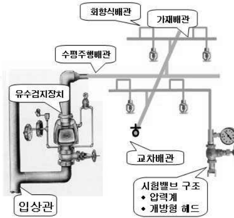
[그림 4-14] 스프링클러설비 배관설치
