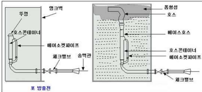
[그림 5-18] 반표면하 방식
