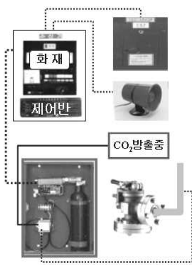
[그림 6-13] 제어반 점검
