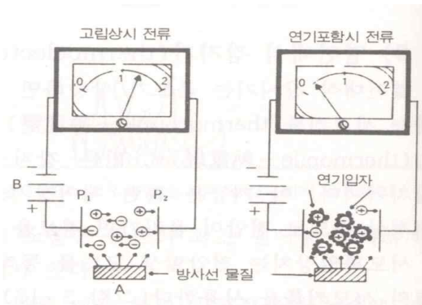
[그림 2-20] 이온화식감지기의 회로구성
