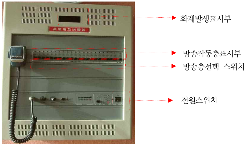
[그림 2-80] 비상방송설비의 스위치 및 표시등
