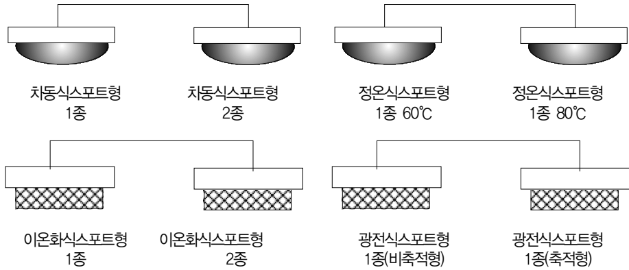
[그림 2-29] 다신호식감지기의 구성
