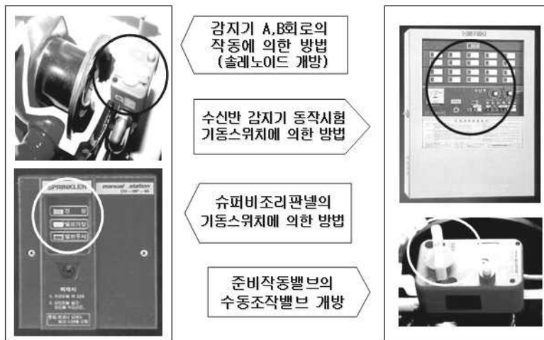
[그림 4-27] 준비작동식 작동방식
