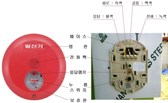
[그림 2-38] 발신기 구성
