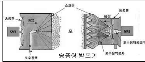
[그림 5-20] 흡출형/송풍형 고발포기
