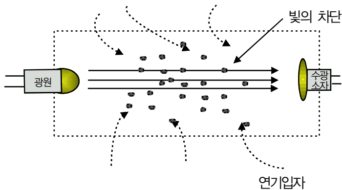
[그림 2-21] 감광식의 감지형태
