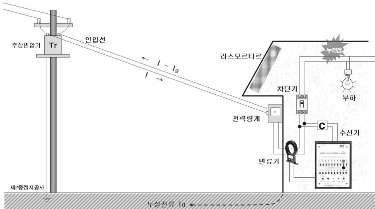
[그림 2-69] 누전경보기 설치구성도
