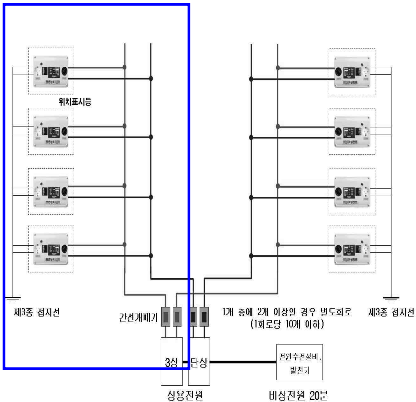
[그림 3-16] 비상콘센트설비의 배선도
