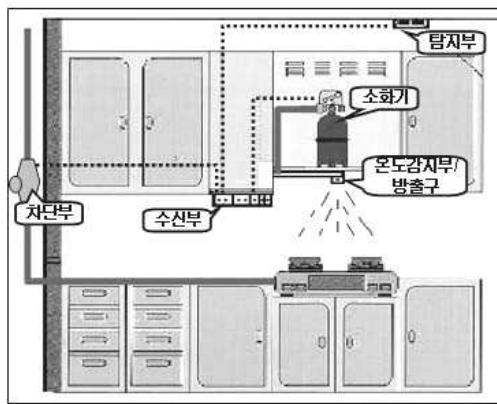
[그림 2-12] 주방용자동소화장치 점검
