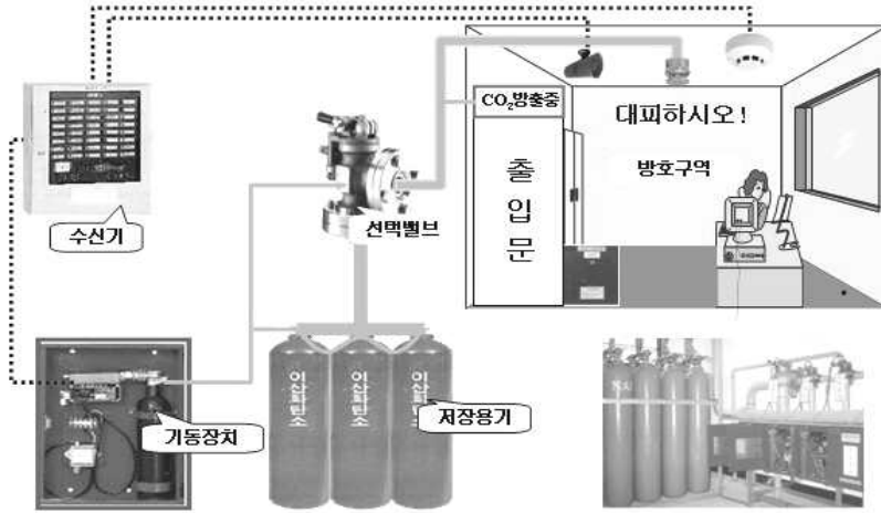
[그림 6-2] 이산화탄소소화설비 구성요소
