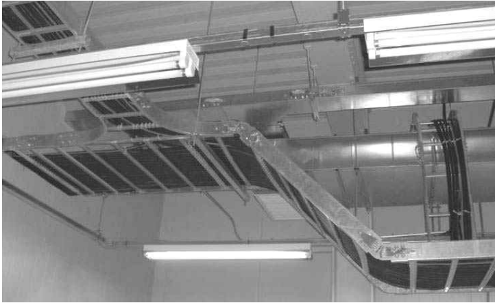
[그림 5-5] 케이블공사
