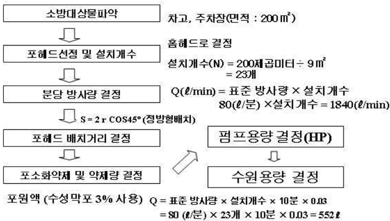
[그림 5-23] 포헤드 설계방식 검토
