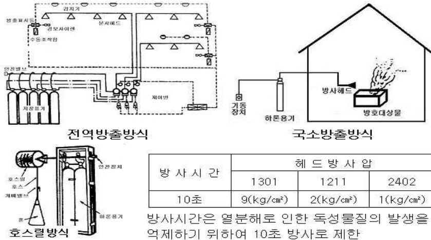
[그림 6-10] 하론약제 방출방식
