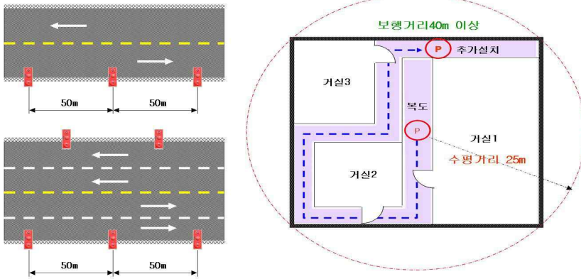
[그림 2-41] 터널 설치기준과 보행거리 초과시 추가설치
