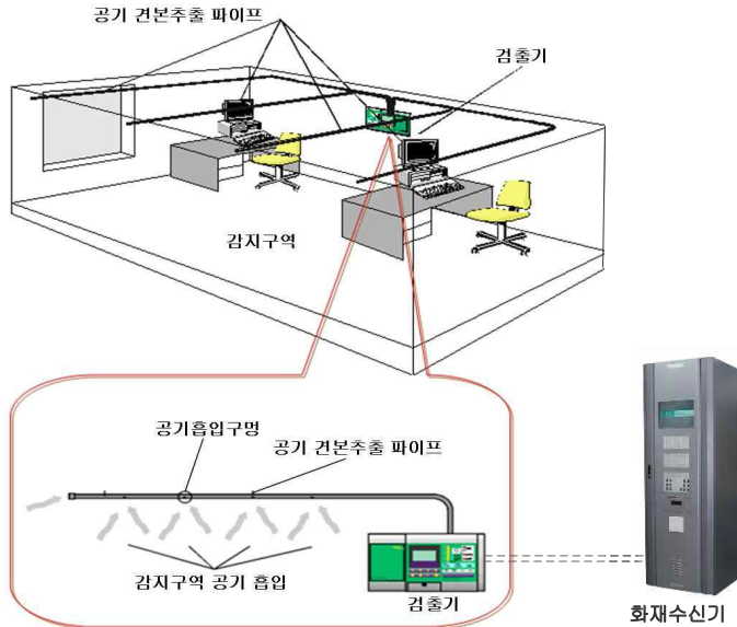
[그림 2-25] 광전식 공기흡입형감지기의 구성
