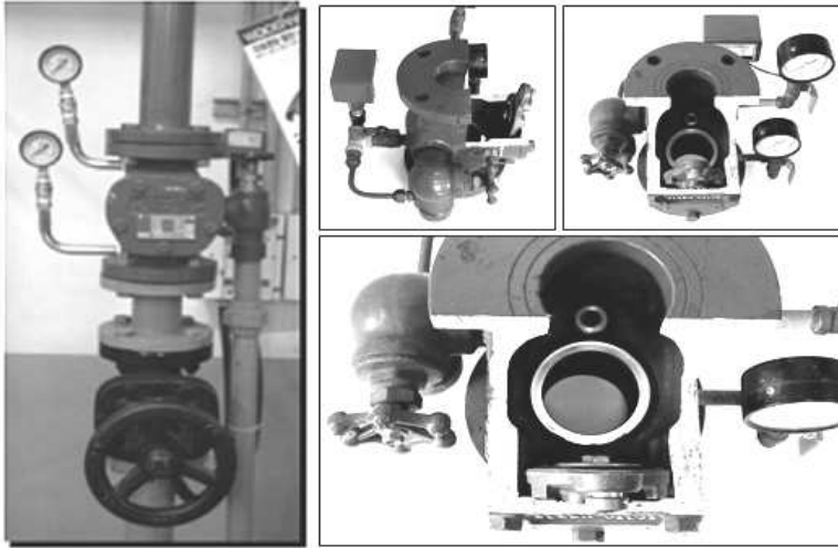
[그림 4-3] 습식밸브 구조
