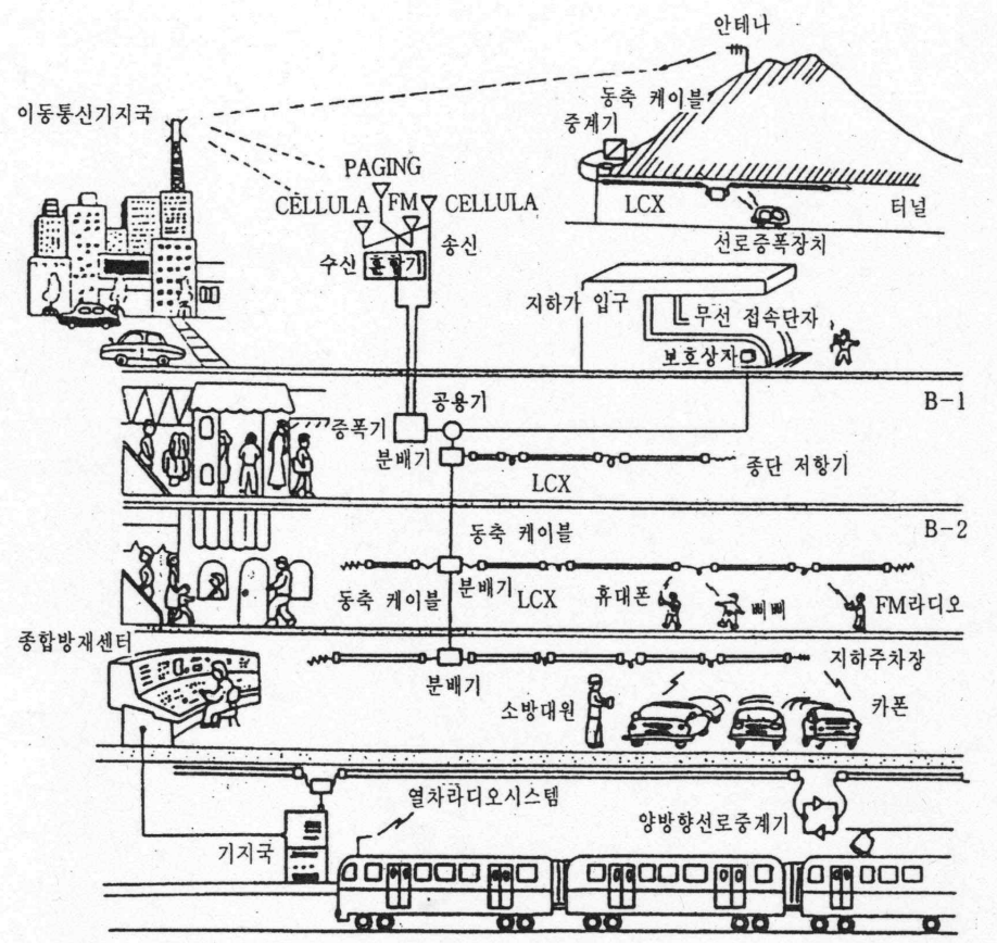
[그림 3-19] 무선통신보조설비의 사용
