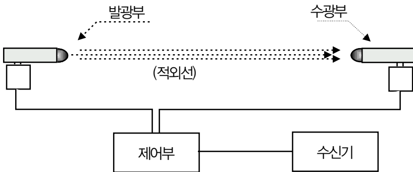
[그림 2-24] 광전식분리형감지기
