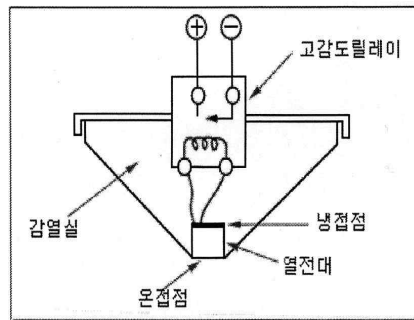
[그림 2-11] 열전대식감지기
