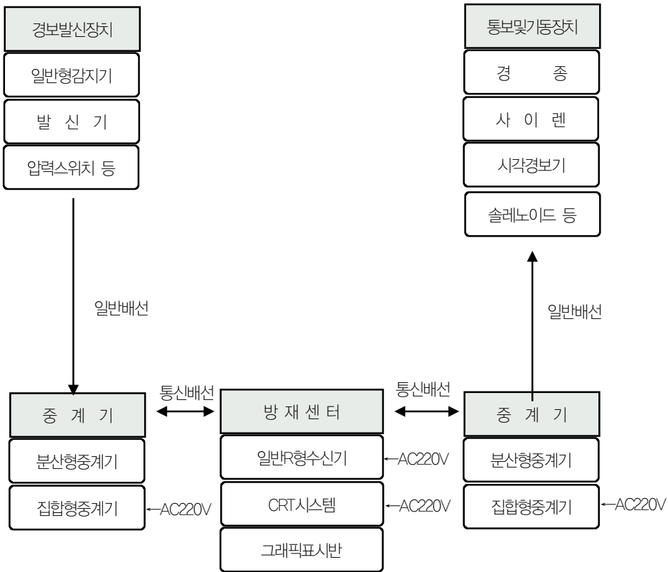
[그림 2-57] 중계기를 사용한 R형 시스템
