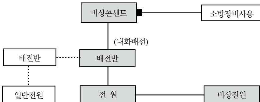
[그림 4-1] 비상콘센트설비의 구성
