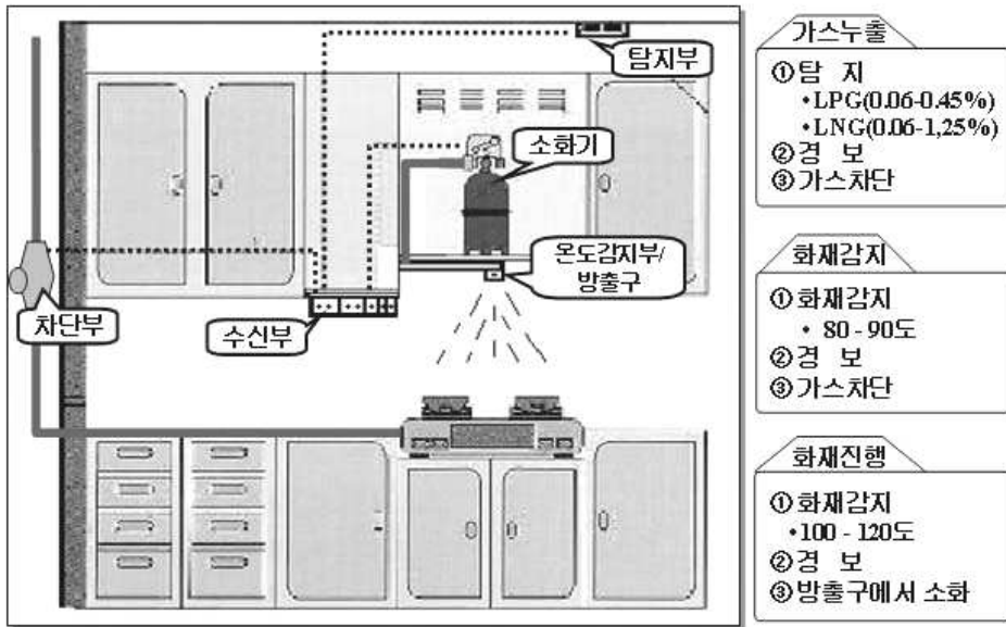
[그림 2-6] 주방용자동소화장치
