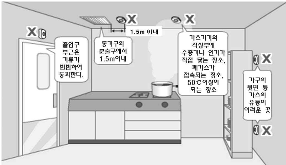
[그림 2-82] 가스누설경보기 검지기 설치장소
