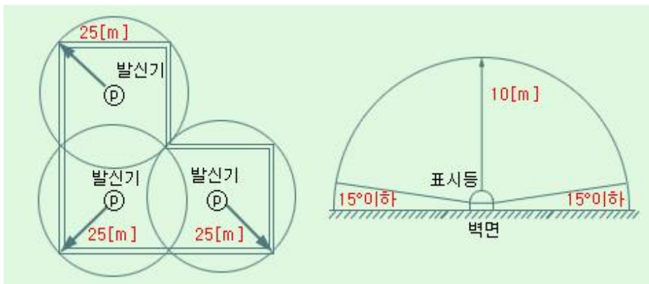
[그림 2-39] 발신기의 설치거리
