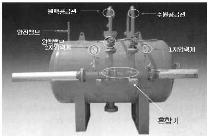
[그림 5-10] 포원액 탱크
