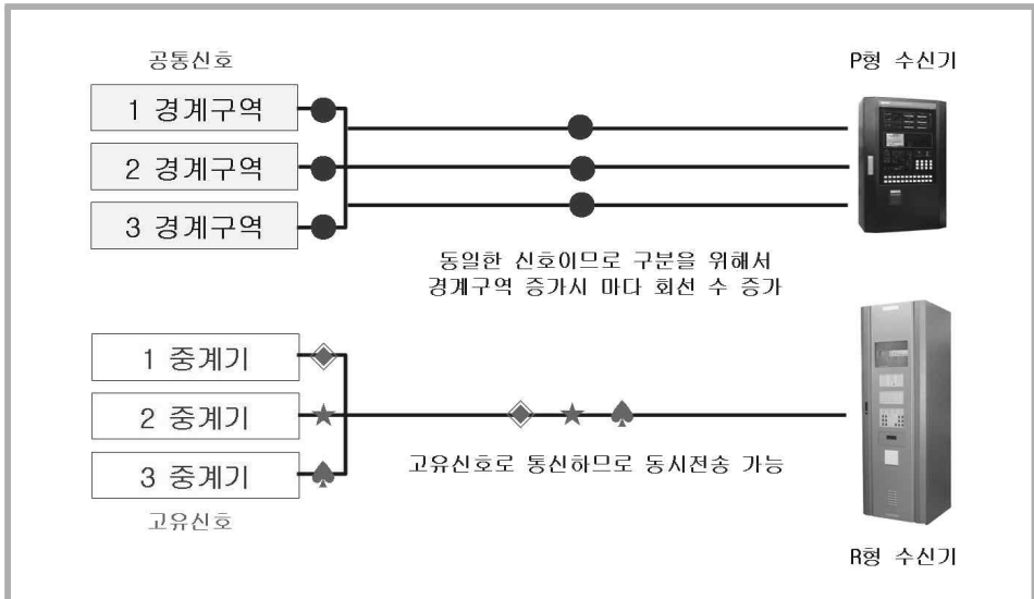
[그림 2-3] 공동신호와 고유신호의 구분
