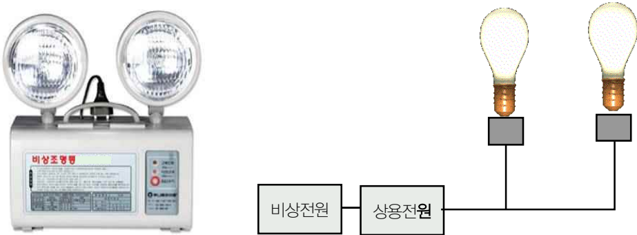
(예비전원을 내장한 비상조명등)
