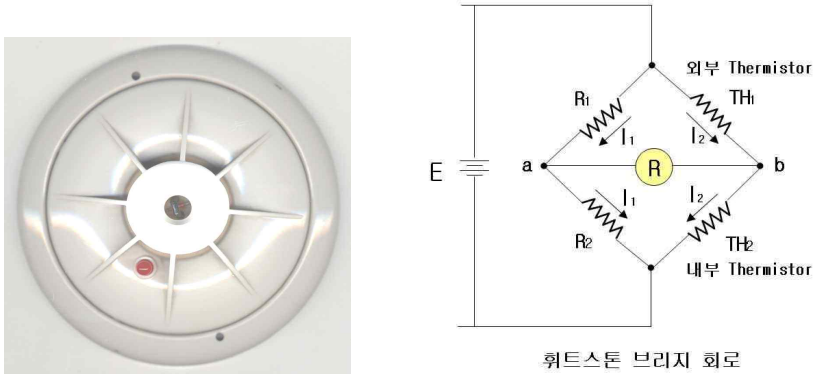
[그림 2-12] 열반도체식감지기
