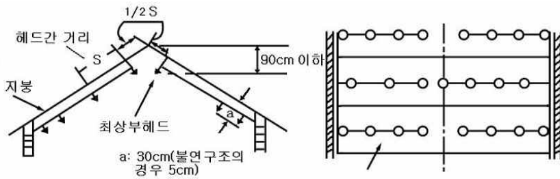
[그림 4-21] 경사지붕의 헤드설치
