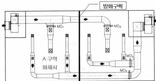
[그림 7-1] 동일실 급배기 방식
