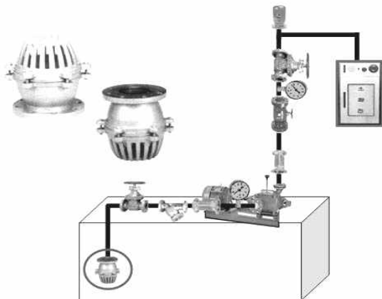
[그림 3-5] 가압송수장치 펌프방식
