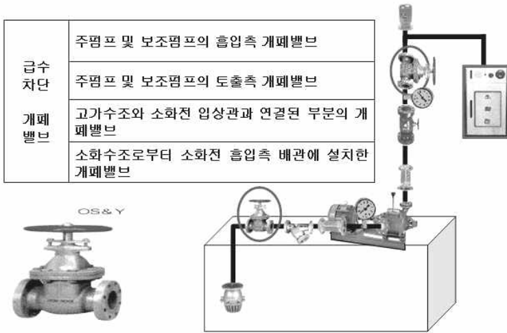
[그림 3-6] 급수차단 밸브 구분
