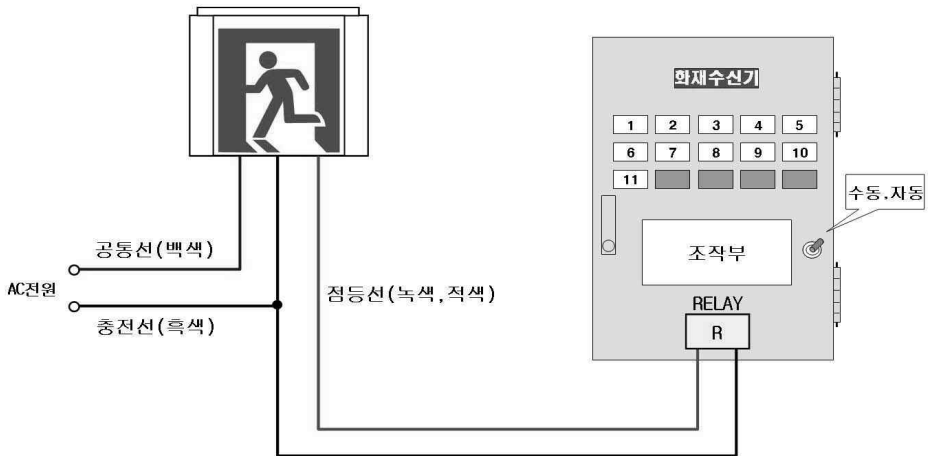
[그림 3-11] 3선식 유도등의 배선
