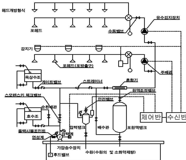
[그림 5-1] 포소화설비 계통도
