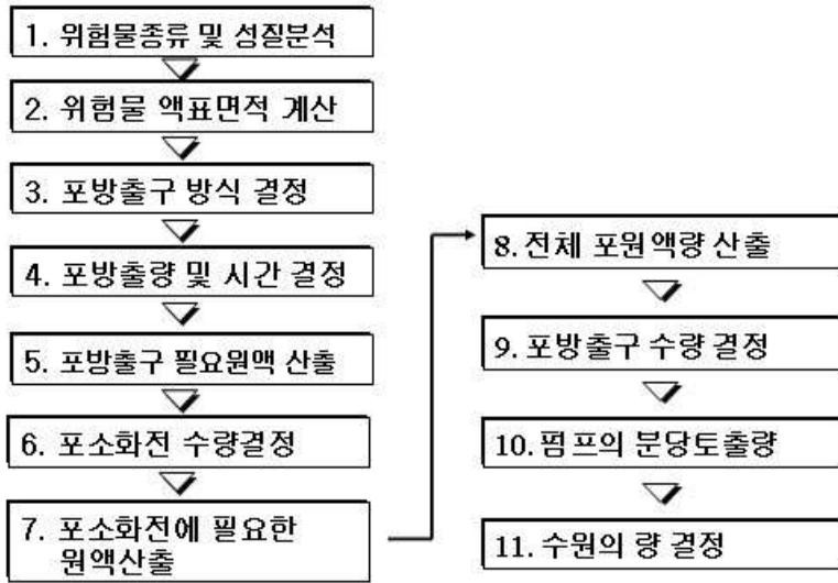
[그림 5-24] 옥외탱크 포소화전설비 설계 검토
