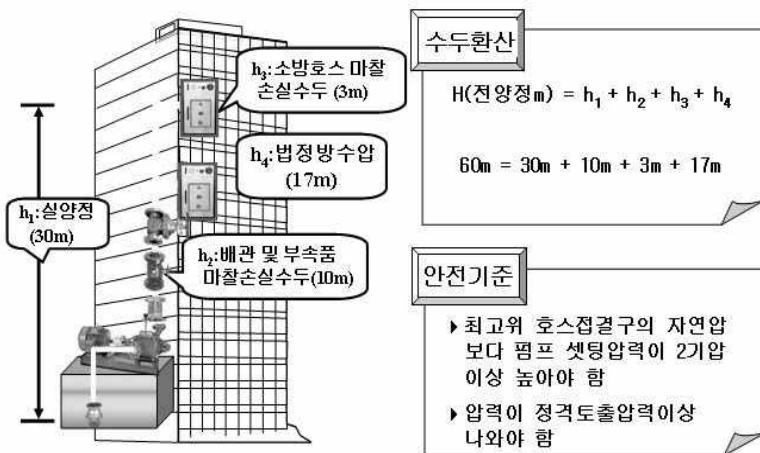
[그림 3-19] 양정계산과 압력설정
