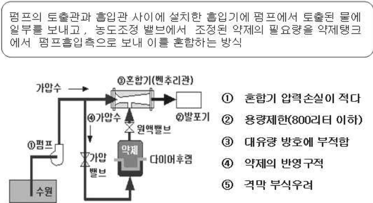
[그림 5-8] 격막이 있는 방식
