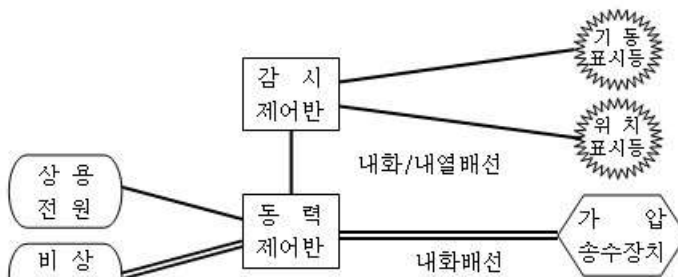
[옥내소화전/SP설비의 배선]
