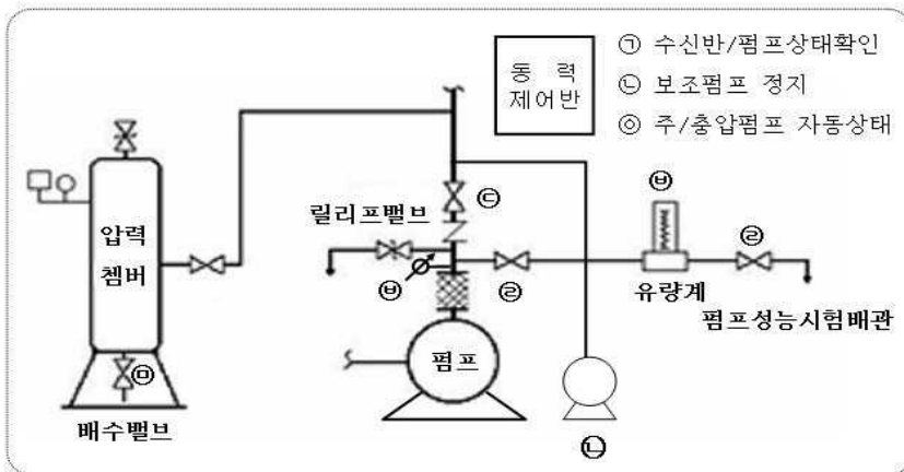
[그림 3-16] 펌프성능시험 방법
