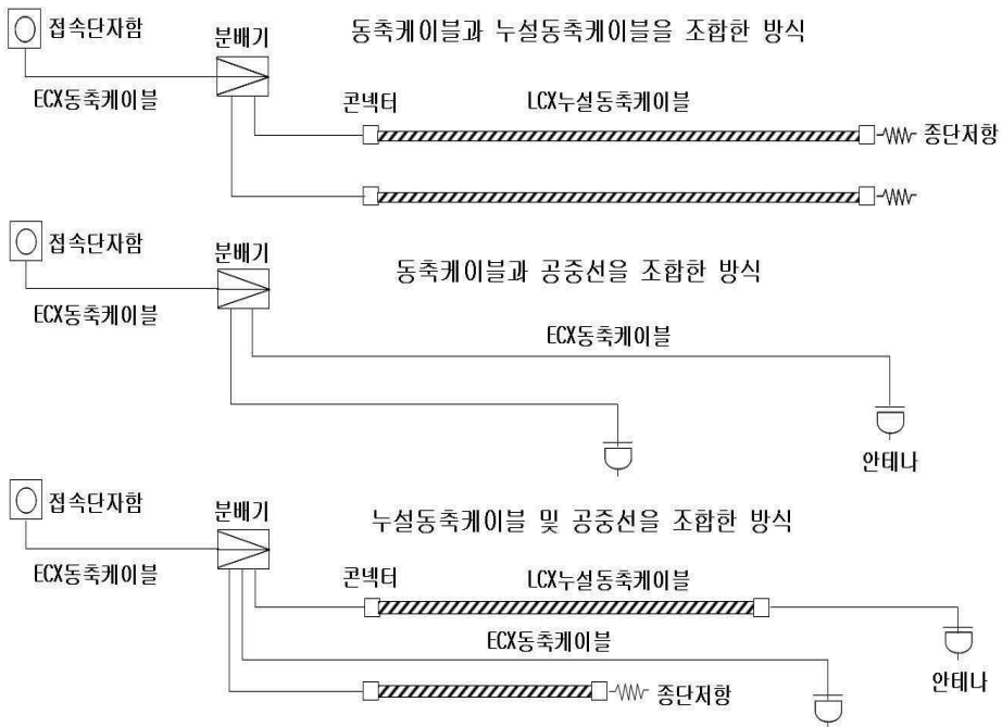
[그림 3-23] 무선통신보조설비의 종류
