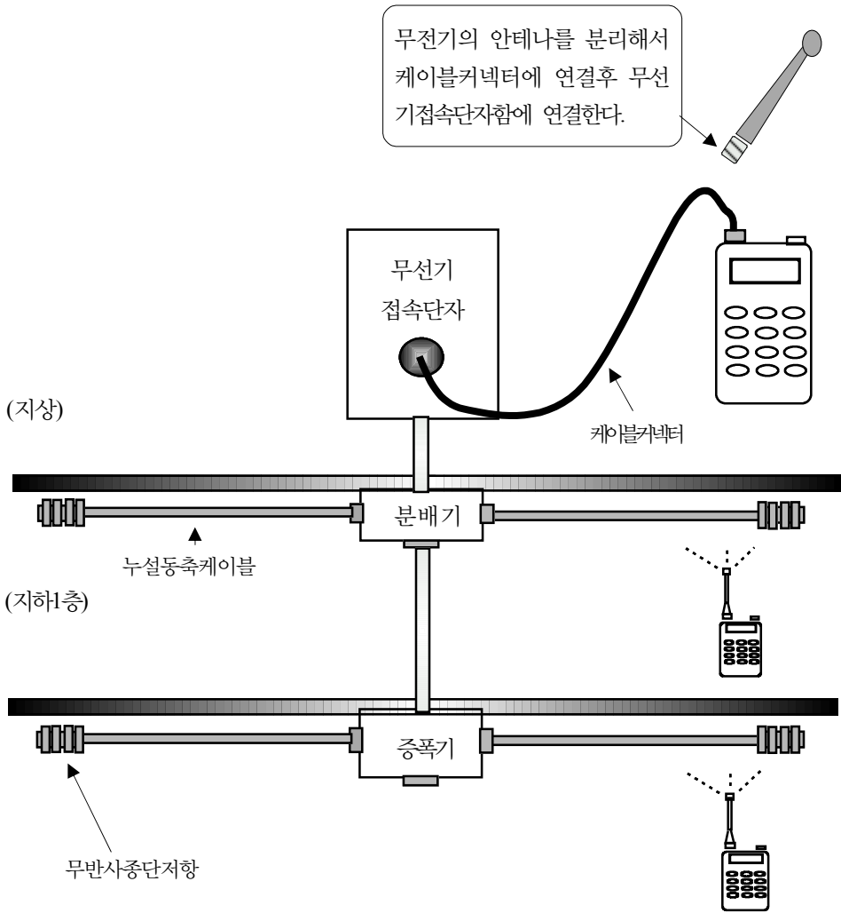
[그림 3-20] 무선통신보조설비의 구성
