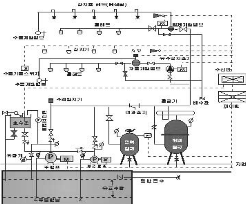
[그림 5-13] 흡헤드설비 방식
