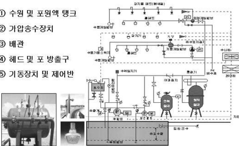
[그림 5-2] 포소화설비 구성요소
