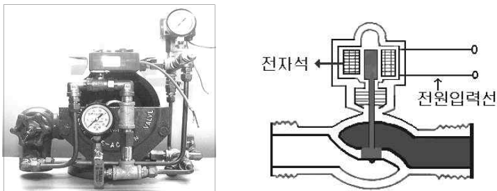
[그림 4-7] 밸브와 솔레노이드
