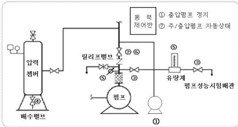
[그림 3-30] 펌프성능시험 방법
