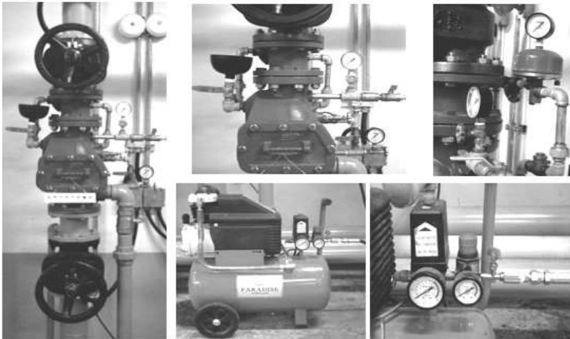
[그림 4-11] 공기압축기와 액셀러레이터
