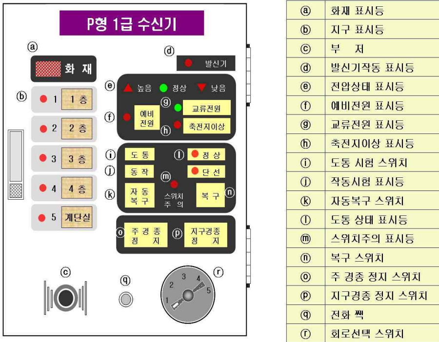
[그림 2-49] P형1급 수신기의 표시등 및 스위치
