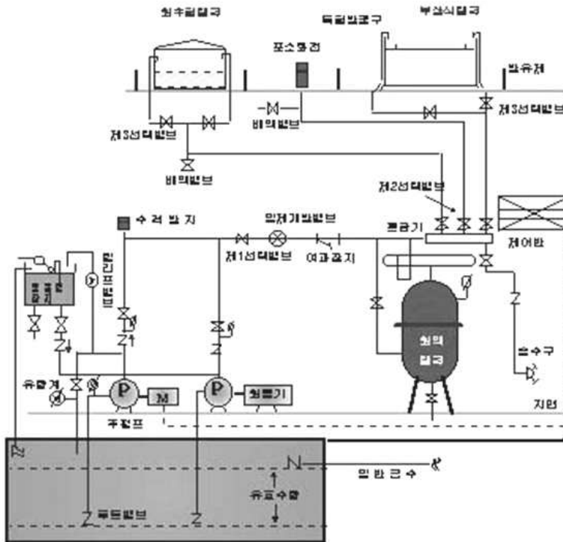
[그림 5-12] 고정포방출설비
