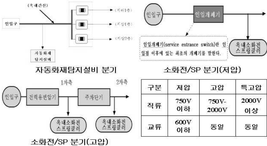
[그림 3-24] 상용전원 분기방식
