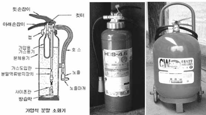
[그림 2-3] 가압식 분말소화기 구조
