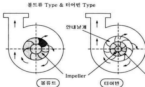
[그림 3-12] 소방용 원심펌프
