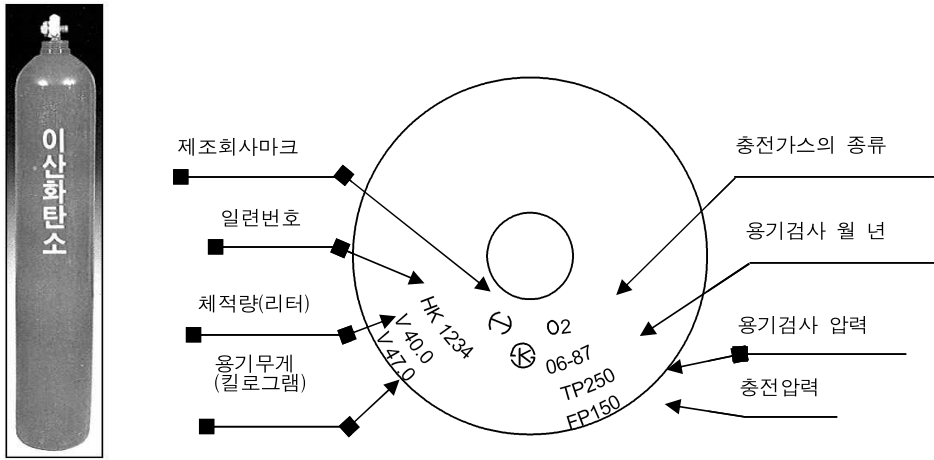
[그림 6-6] 가스저장용기
