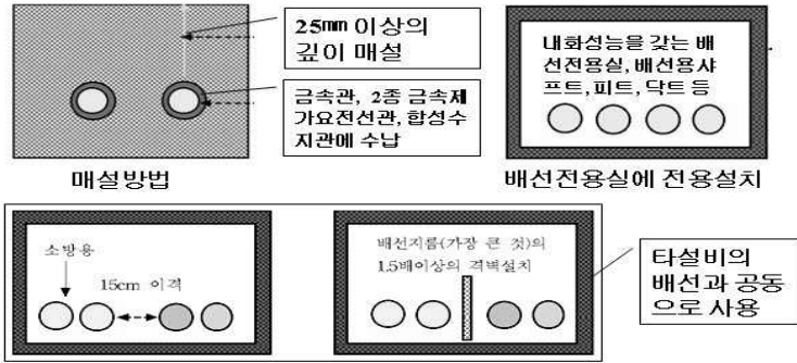
[그림 3-25] 내화배선 공사방법
