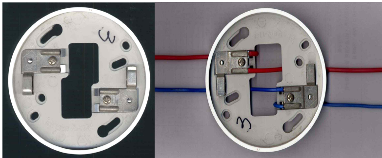
[그림 2-8] 감지기 베이스 및 배선방법
