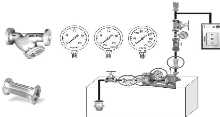
[그림 3-7] 흡입측 배관 부속품 및 밸브류
