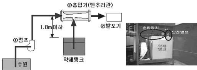
[그림 5-6] 라인프로포셔너 방식
