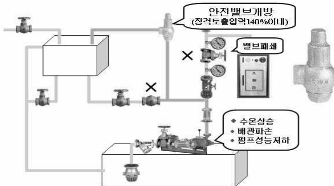
[그림 3-11] 순환배관 구조와 기능
