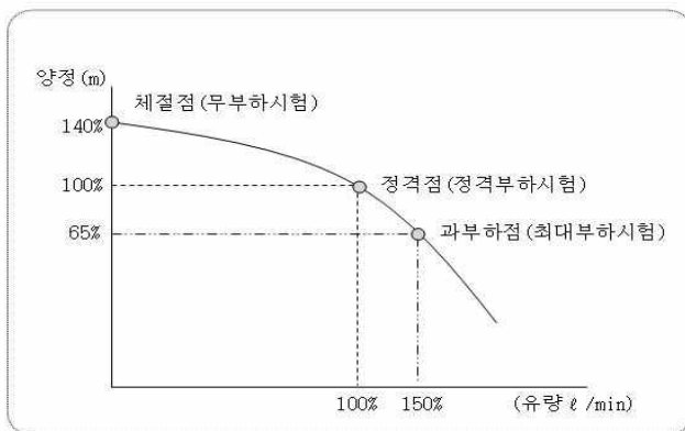
[소방펌프의 특성곡선]
