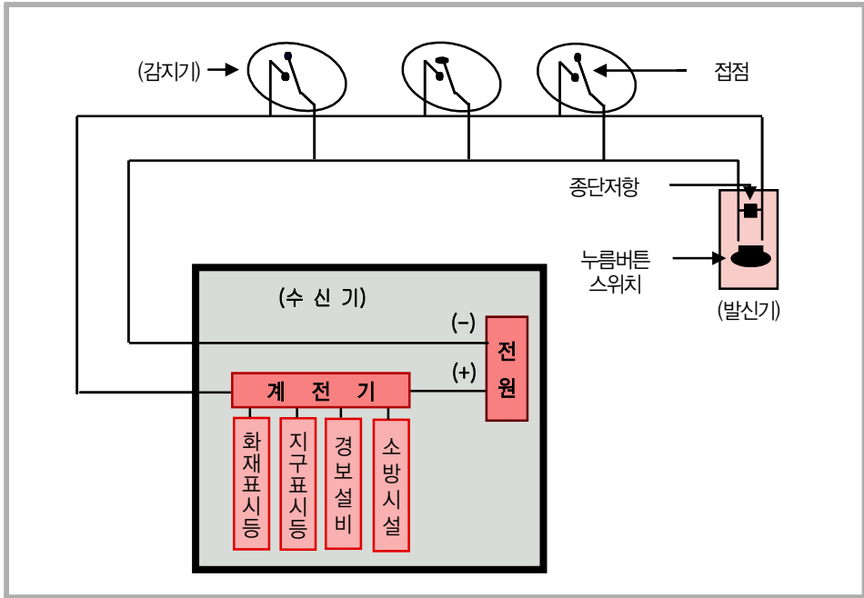
[그림 2-2] 자동화재탐지설비의 회로 간략도
