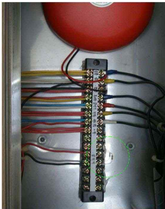
[그림 2-52] 종단저항 설치(발신기세트함 및 종단감지기)
