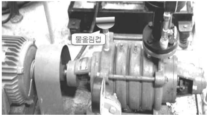
[그림 3-31] 후트밸브 고장여부 점검
