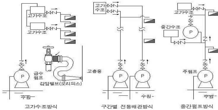
[그림 3-21] 감압방식
