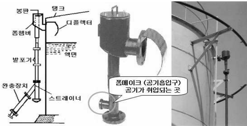
[그림 5-15] II형 방출구
