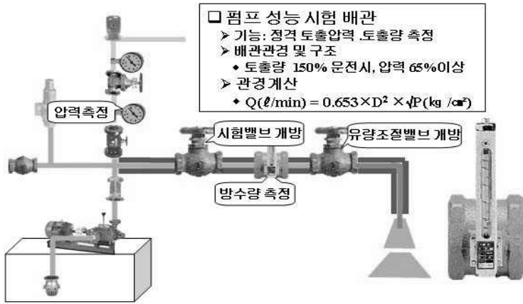
[그림 3-15] 펌프성능시험 배관
