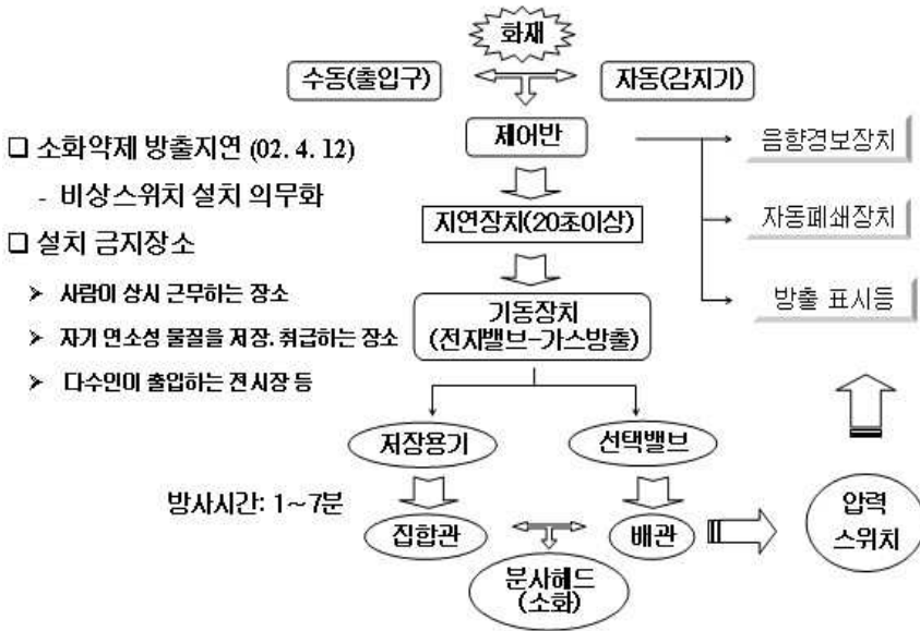
[그림 6-7] 이산화탄소설비 작동원리 요약
