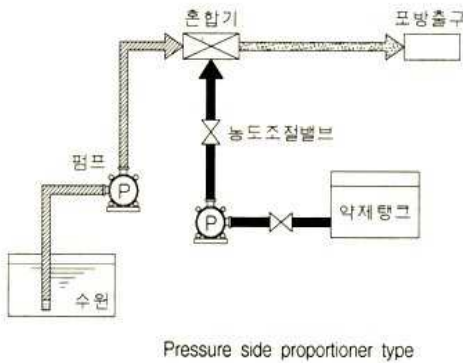
[그림 5-11] 프레저사이드프로포셔너 방식
