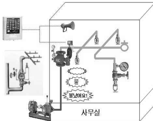
[그림 4-2] 스프링클러설비 구조 및 작동
