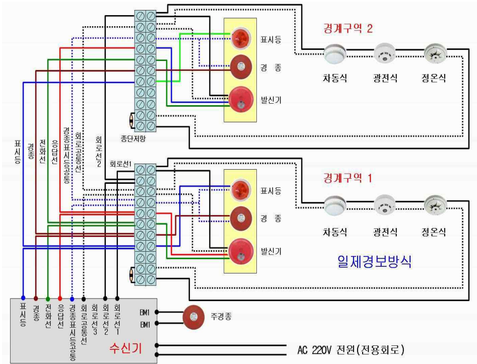
[그림 2-54] 여러 경계구역의 연결
