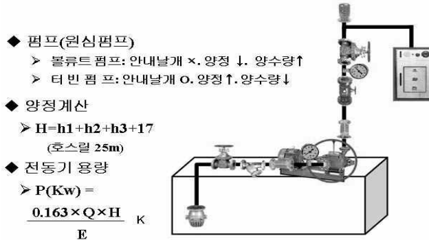
[그림 3-13] 펌프방식의 전동기 용량
