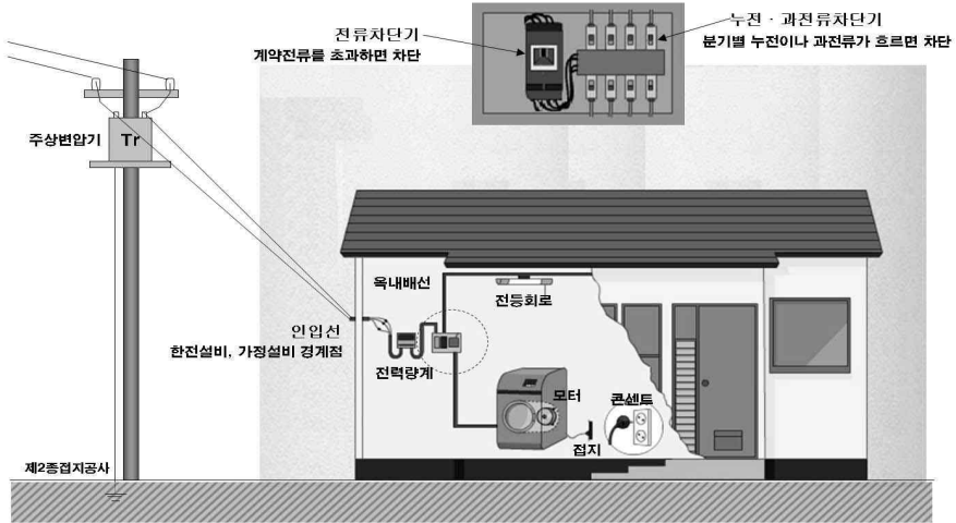
[그림 5-1] 일반주택의 옥내·외 배선
