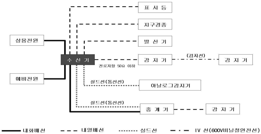
[그림 5-7] 자동화재탐지설비 구간배선
