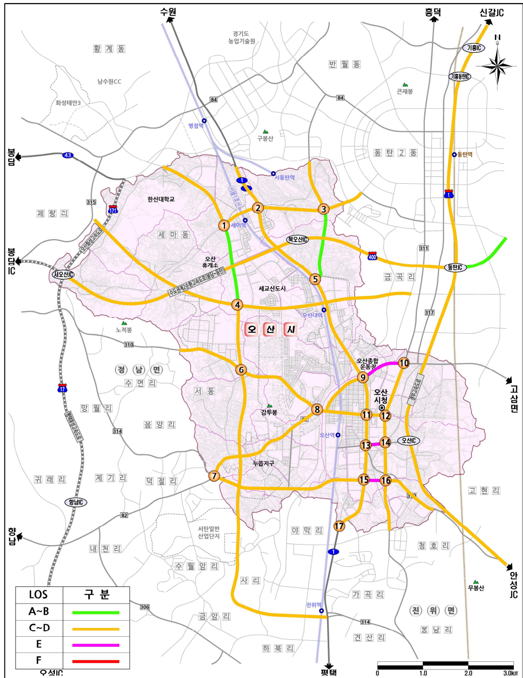
〈 장래 개선안 시행시 주요가로 교통소통 분석결과(2035년) 〉
