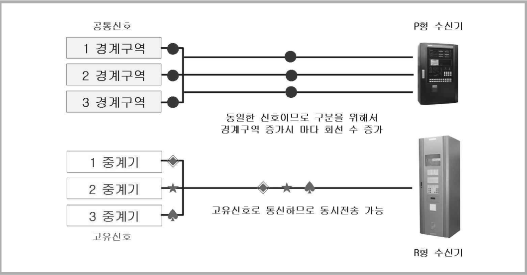
[그림 2-3] 공통신호와 고유신호의 구분
