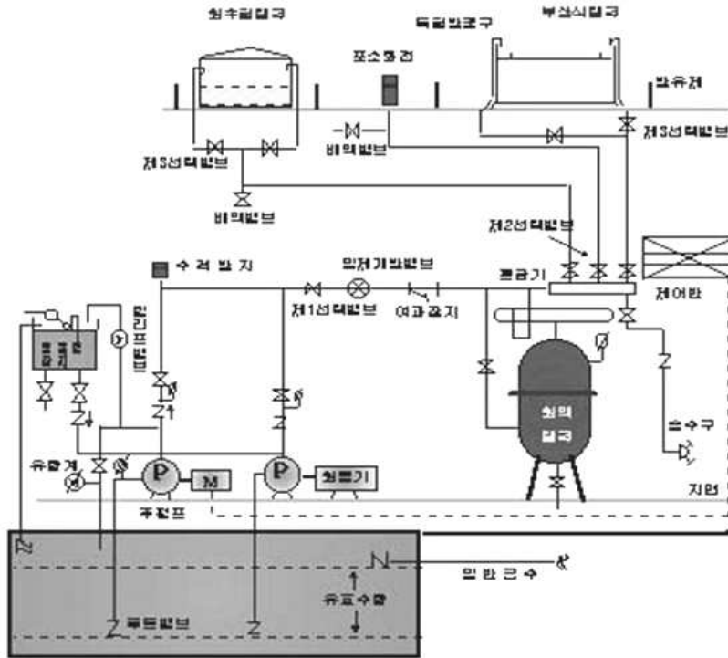
[그림 5-12] 고정포방출설비
