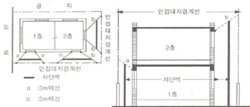
[그림 3-4] 차단벽 설치
