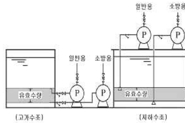
[그림 3-3] 유효수량 산정
