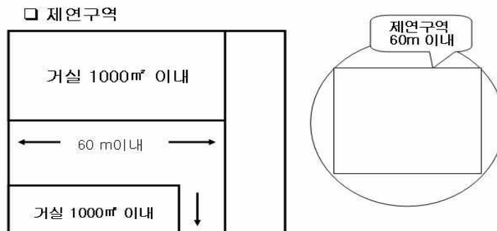
[그림 7-5] 제연구역 설정
