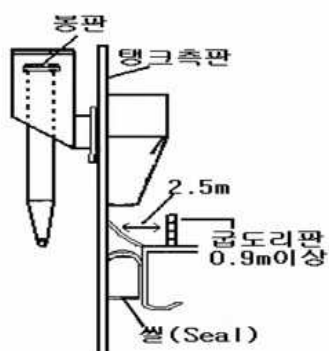
[그림 5-16] 특형 방출구
