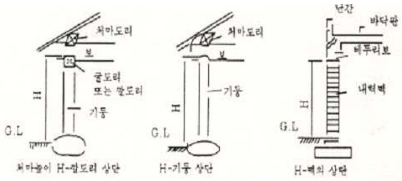
[그림 2-14] 처마높이 산정
