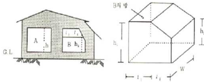
[그림 2-13] 반자 높이 산정
