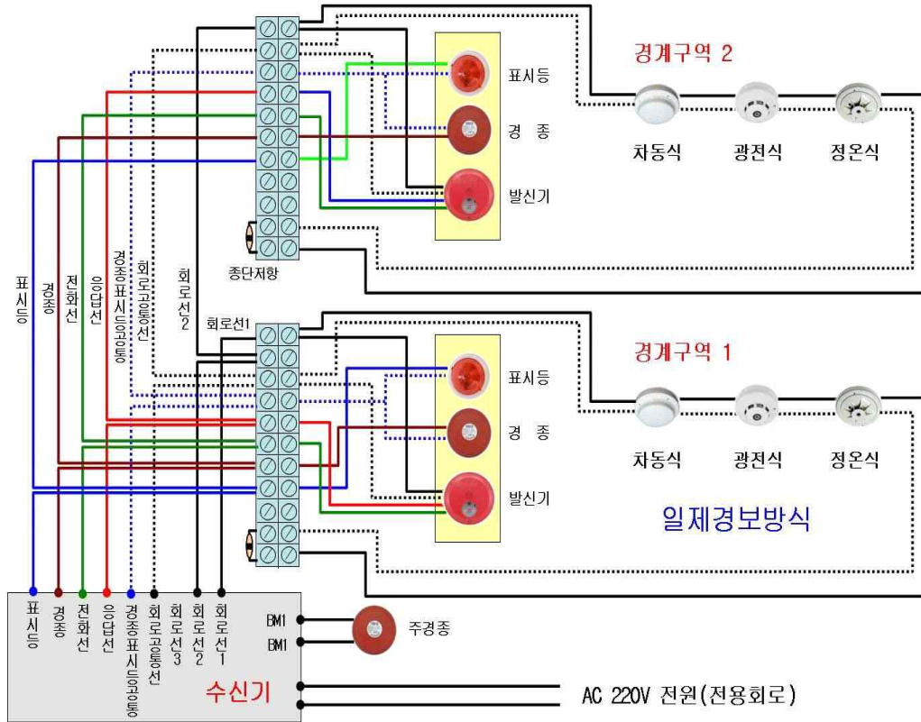
[그림 2-54] 여러 경계구역의 연결
