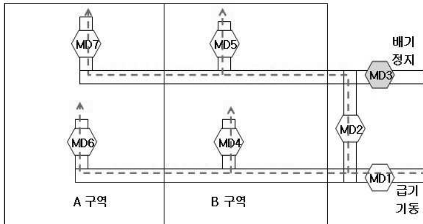
[그림 7-3] 평상시 공기조화설비 기능
