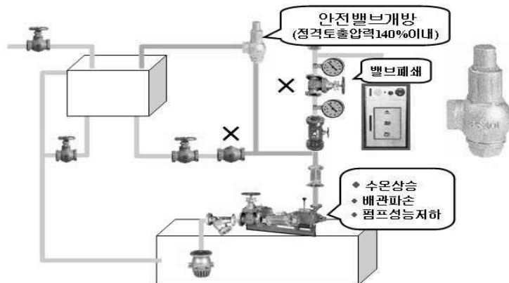
[그림 3-11] 순환배관 구조와 기능
