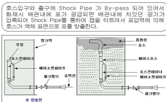
[그림 5-18] 반표면하 방식
