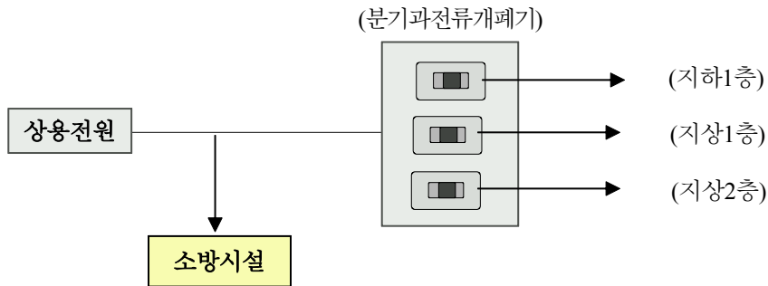
[그림 5-3] 소방시설 상용전원의 분기(○)
