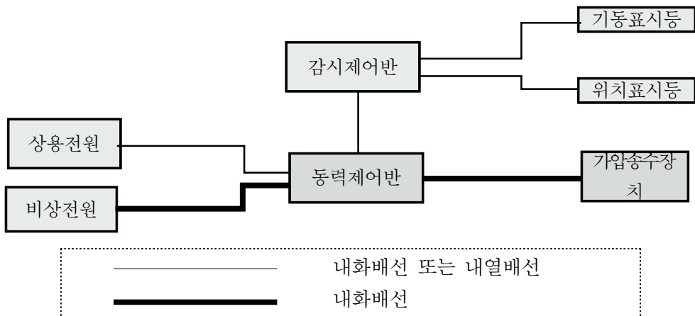
[그림 5-8] 소화전 구간배선
