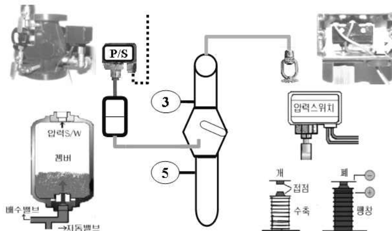
[그림 4-4] 압력스위치와 리타딩챔버
