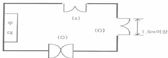
[그림 4-5] 출구의 문 설치기준
