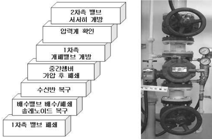
[그림 4-29] 준비작동식 복구순서
