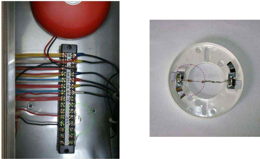
[그림 2-52] 중단저항 설치(발신기세트함 및 중단감지기)
