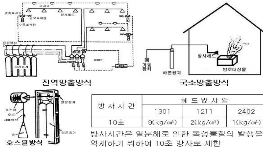
[그림 6-10] 하론약제 방출방식
