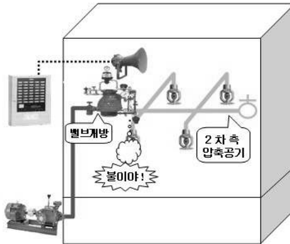
[그림 4-9] 건식스프링클러설비 구성
