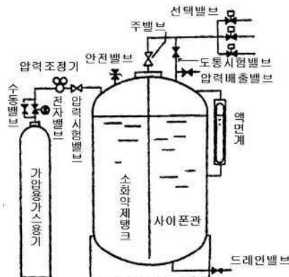
[그림 6-9] 가압식 저장방식
