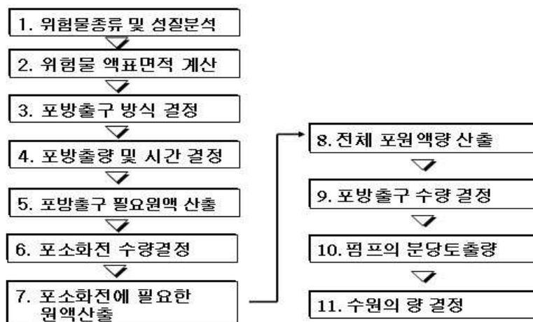
[그림 5-24] 옥외탱크 포소화전설비 설계 검토
