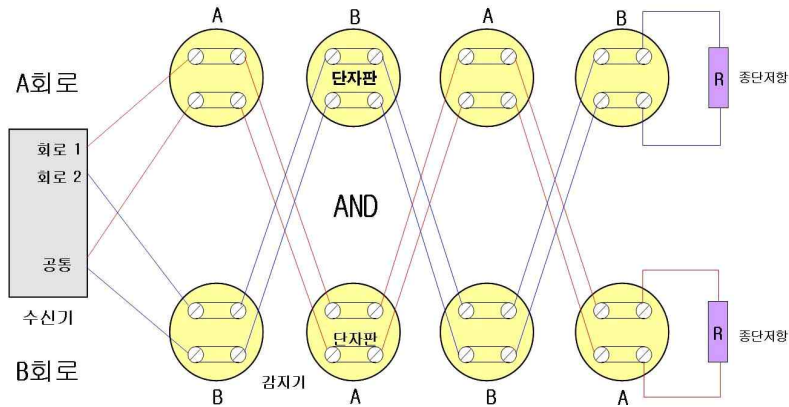
[그림 2-46] 자동소화설비 화재감지기용 회로는 교차회로
