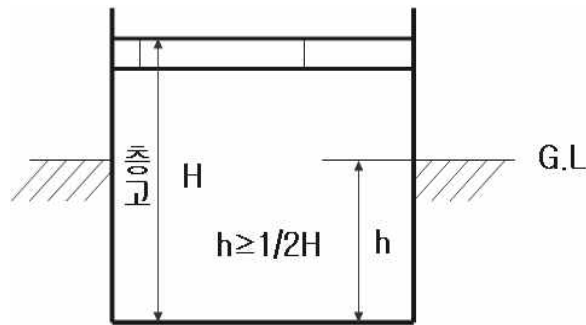
[그림 1-1] 지 하 층
