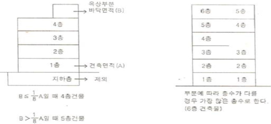
[그림 2-15] 건축물의 층수산정
