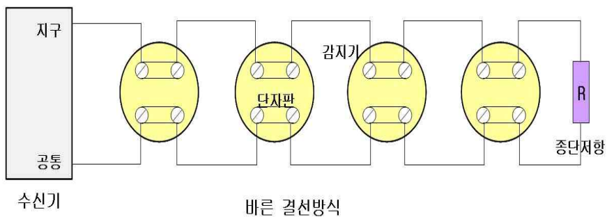
[그림 2-53] 감지기 배선 송배선방식
