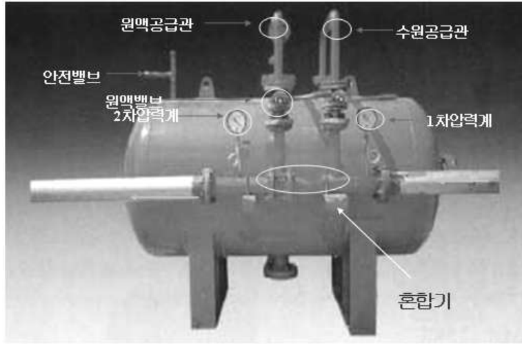
[그림 5-10] 포원액 탱크
