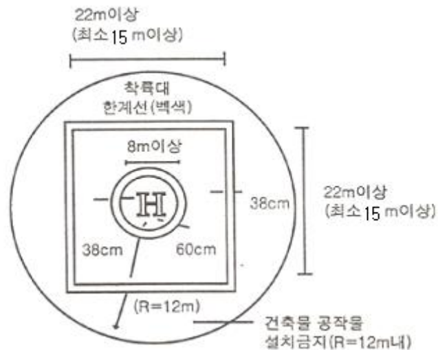
[그림 4-15] 헬리포트의 설치기준
