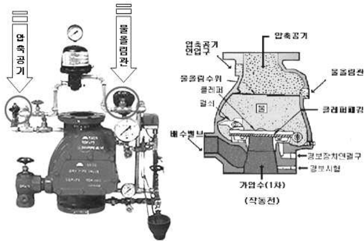
[그림 4-10] 건식밸브 구조
