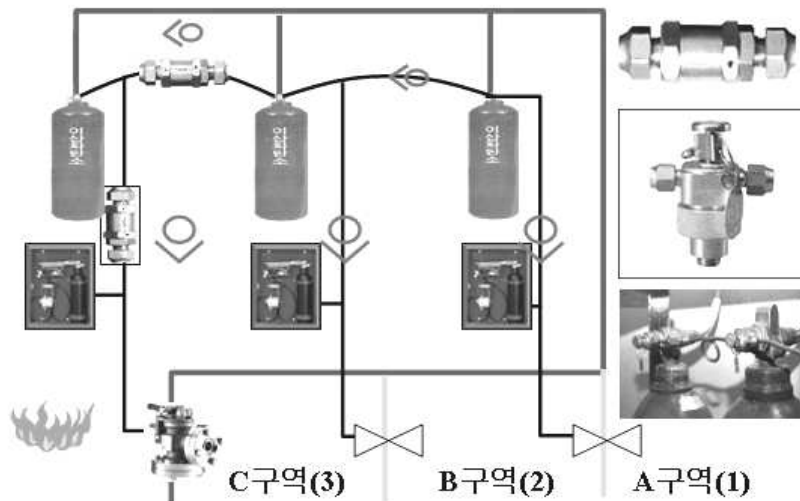
[그림 6-3] 방호구역과 선택밸브
