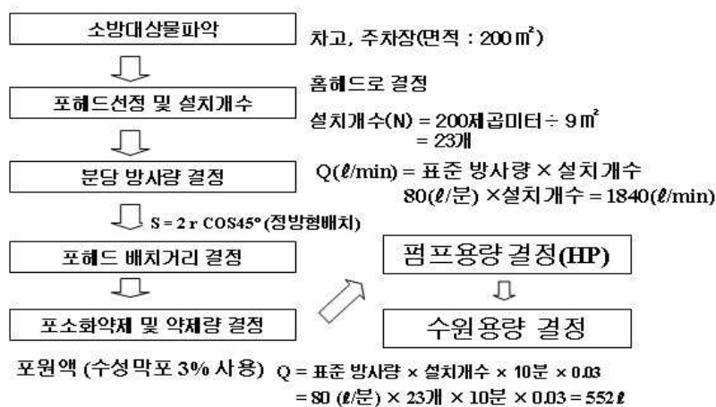
[그림 5-23] 포헤드 설계방식 검토
