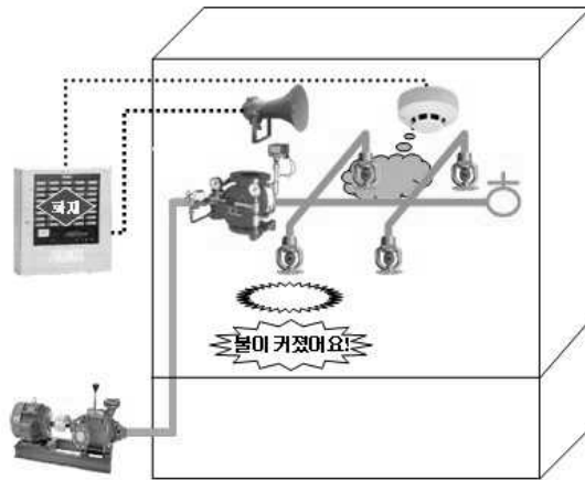
[그림 4-5] 준비작동식 구조
