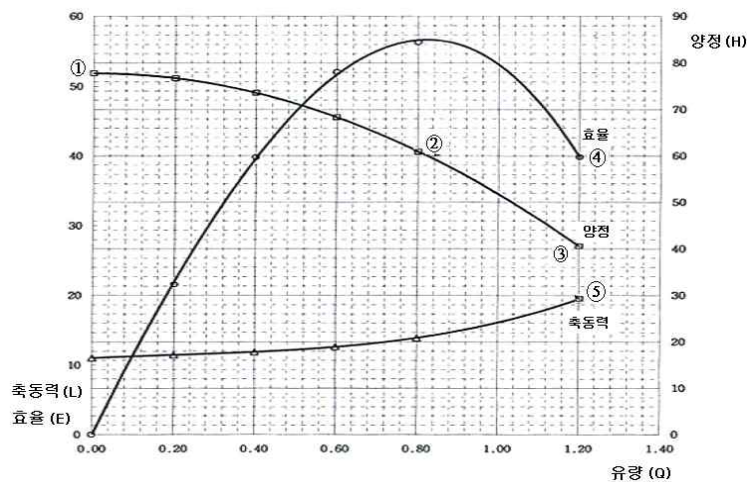
[그림 3-20] 양정계산과 압력셋팅
