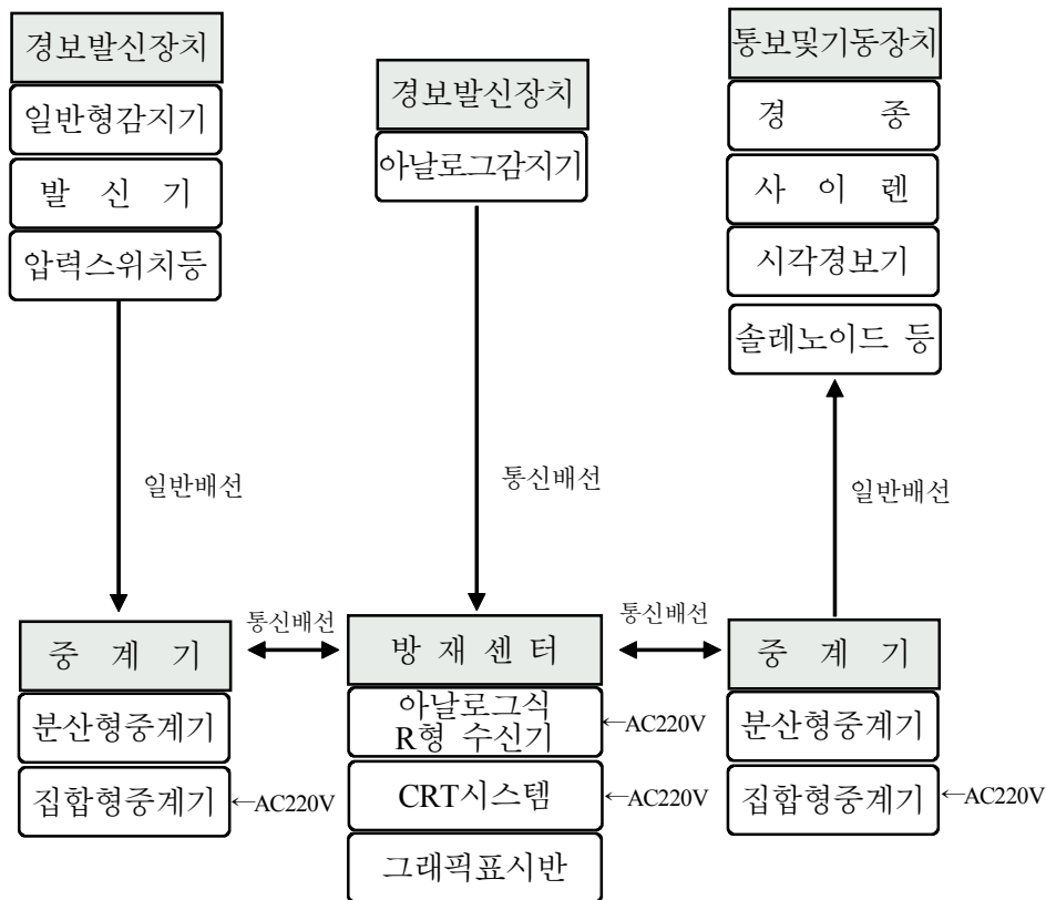
[그림 2-58] 아날로그식 감지기를 사용하는 경우
