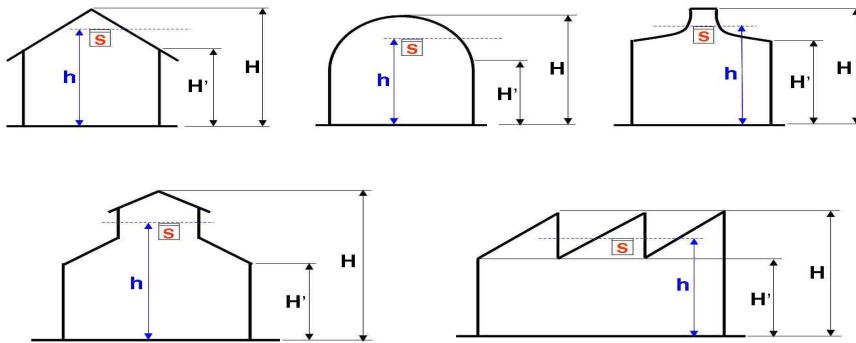
[그림 2-31] 건축물별 감지기의 설치높이 산정방법
