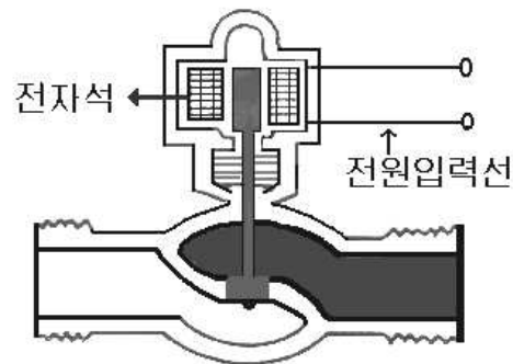
[그림 4-7] 밸브와 솔레노이드
