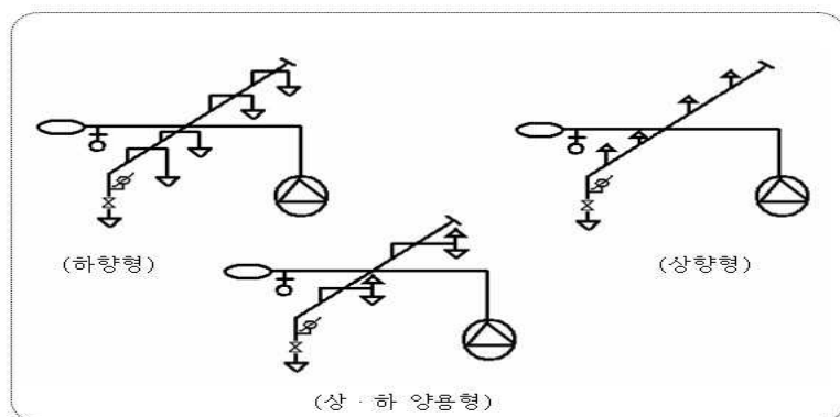
[그림 4-17] 헤드설치방법
