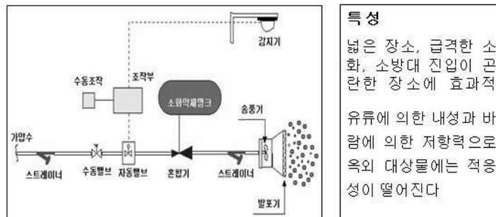
[그림 5-19] 고발포형 고정포 방출구
