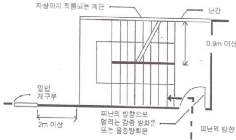
[그림 4-13] 옥외피난계단의 구조
