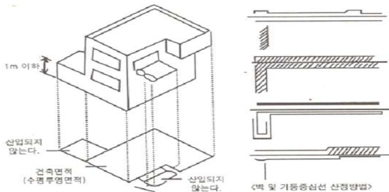
[그림 2-4] 건축면적의 산정방법
