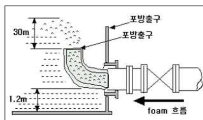
[그림 5-17] 표면하 주입구
