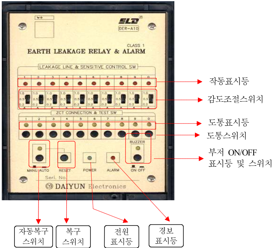
[그림 2-71] 누전경보기의 표시등 및 스위치
