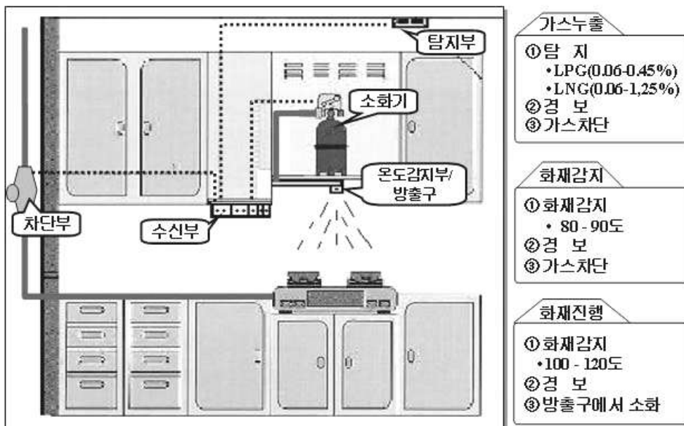
[그림 2-6] 주방용자동소화장치
