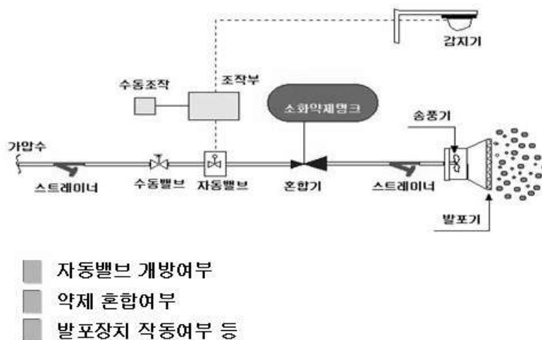
[그림 5-26] 고발포형 고정포 방출구 점검
