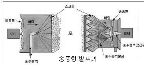
[그림 5-20] 흡출형/송풍형 고발포기
