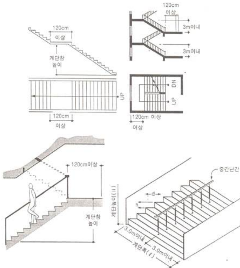
[그림 4-9] 계단의 설치기준
