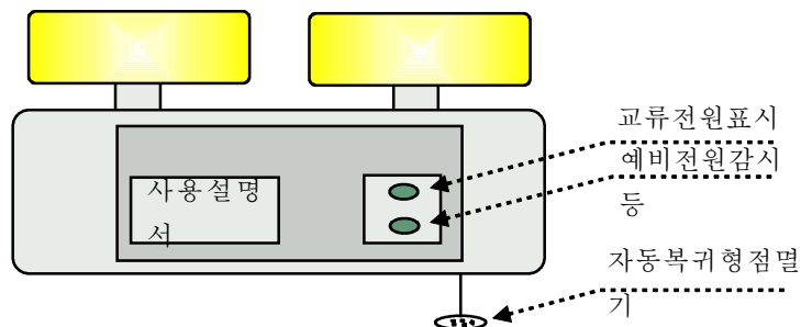
[그림 3-15] 비상조명등 표시등 및 스위치
