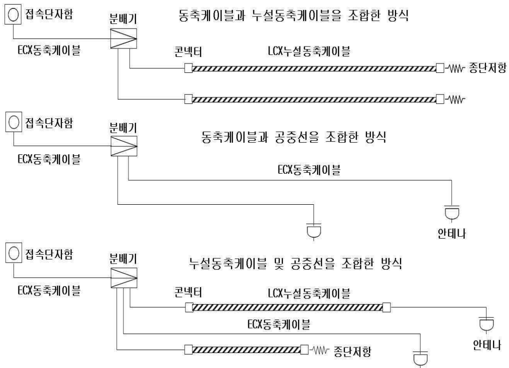
[그림 3-23] 무선통신보조설비의 종류
