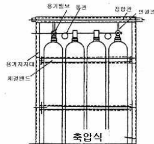
[그림 6-8] 축압식 저장방식
