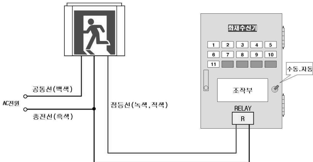
[그림 3-11] 3선식 유도등의 배선
