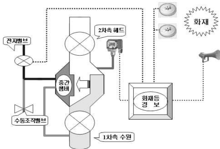
[그림 4-6] 준비작동식밸브 교차회로방식
