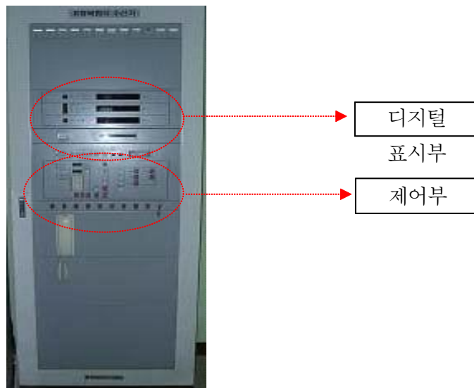
[그림 2-61] R형 수신기의 표시장치 및 제어부
