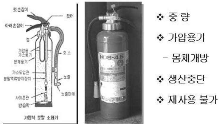
[그림 2-8] 가압식 분말소화기 점검
