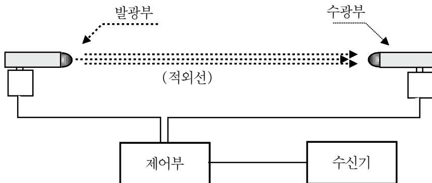
[그림 2-24] 광전식분리형감지기
