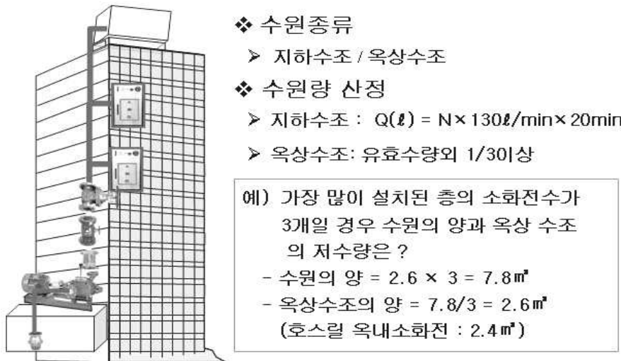
[그림 3-2] 옥내소화전 수원산정
