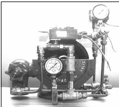
[그림 4-7] 밸브와 솔레노이드
