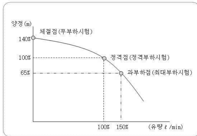
[소방펌프의 특성곡선]
