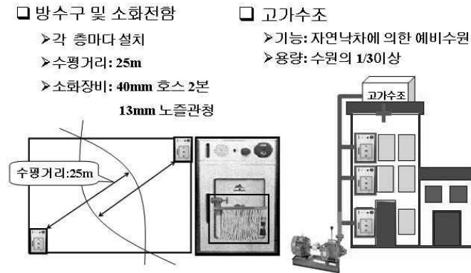
[그림 3-18] 소화전함 설치
