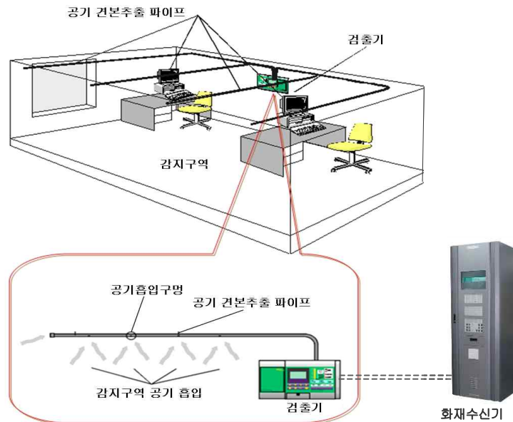
[그림 2-25] 광전식 공기흡입형감지기의 구성
