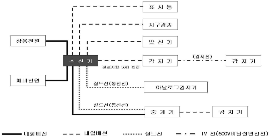
[그림 5-7] 자동화재탐지설비 구간배선
