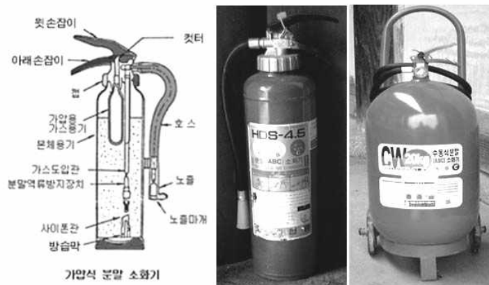
[그림 2-3] 가압식 분말소화기 구조
