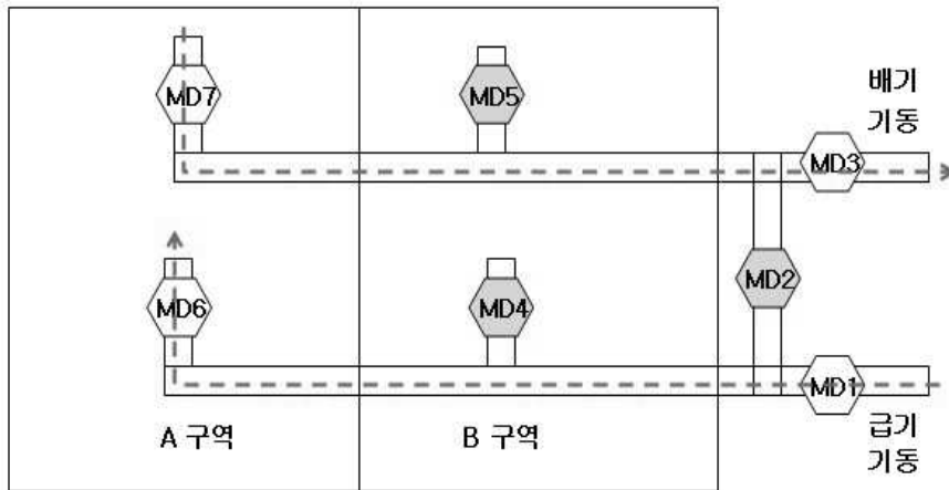
[그림 7-4] 화재시 제연설비로 전환
