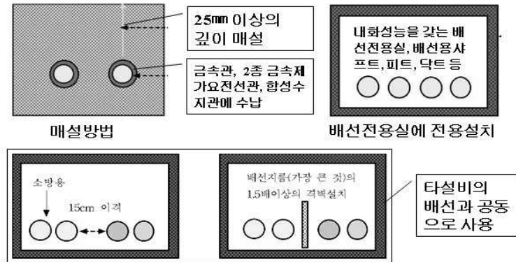
[그림 3-25] 내화배선 공사방법
