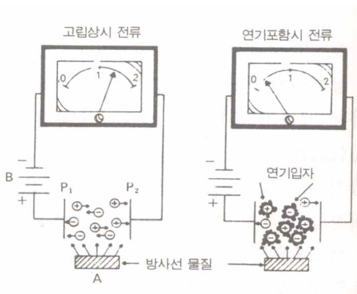
[그림 2-20] 이온화식감지기의 회로구성
