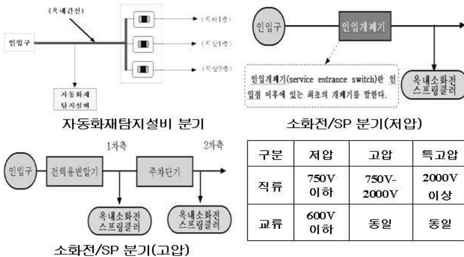
[그림 3-24] 상용전원 분기방식
