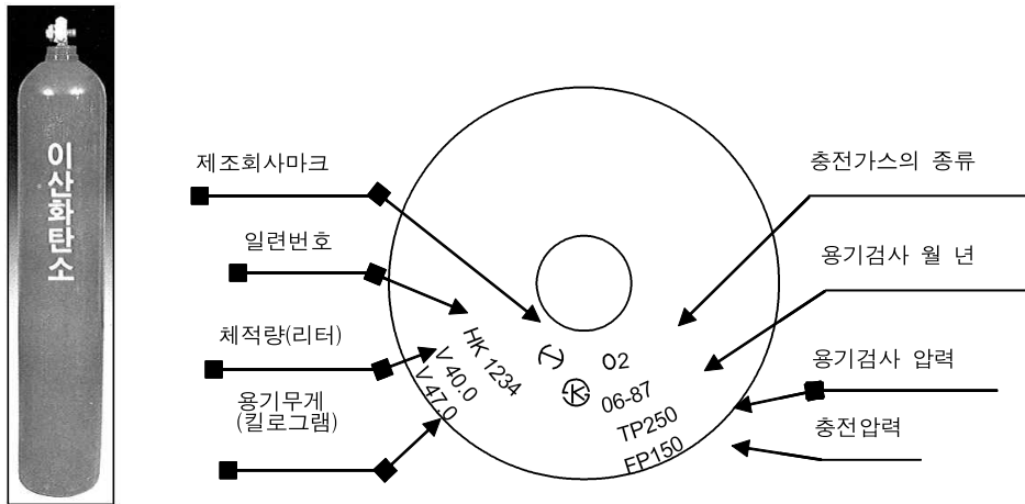
[그림 6-6] 가스저장용기
