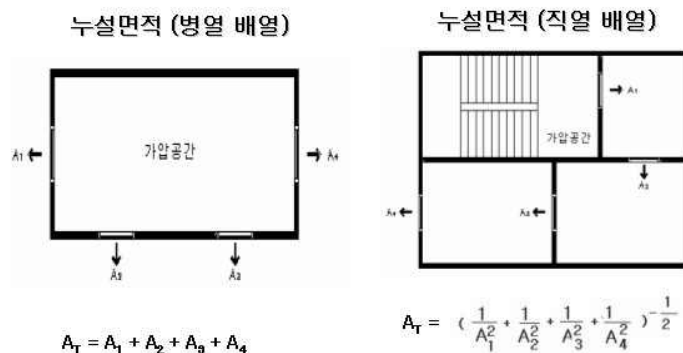
[그림 7-6] 누설면적 계산
