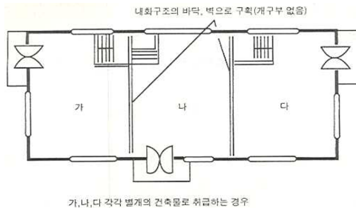
[그림 4-1] 별개의 건축물
