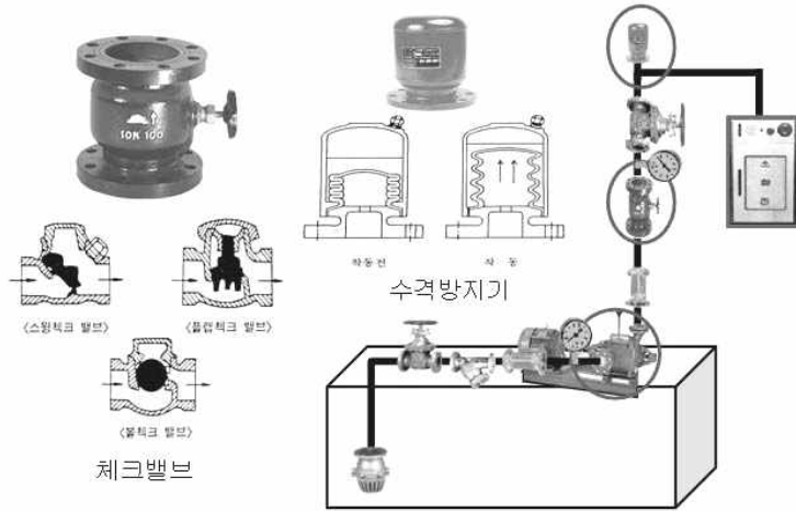
[그림 3-8] 체크밸브와 수격방지기
