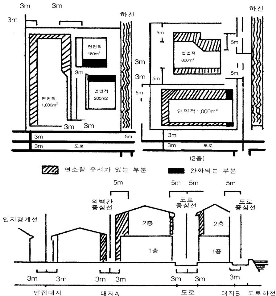
[그림 1-2] 연소할 우려가 있는 부분
