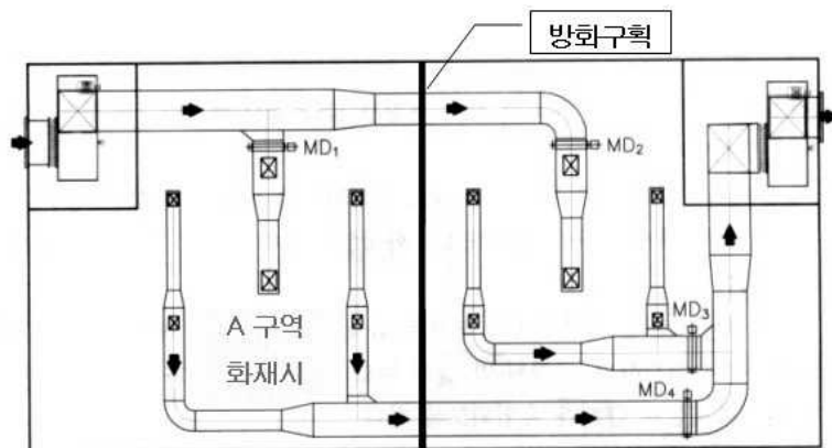
[그림 7-1] 동일실 급배기 방식
