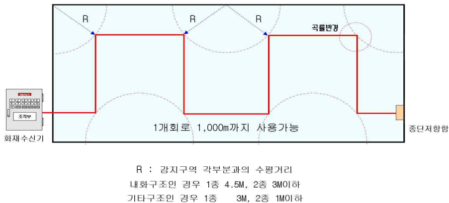
[그림 2-35] 정온식감지선형감지기 설치기준
