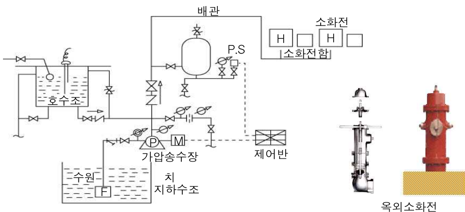
[그림 3-29] 옥외소화전 계통도
