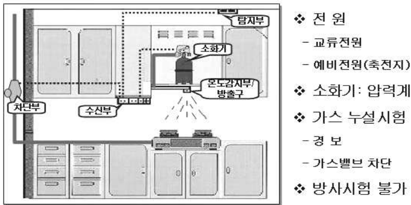
[그림 2-12] 주방용자동소화장치 점검
