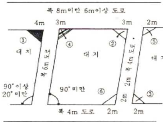
[그림 2-3] 가각정리의 예시
