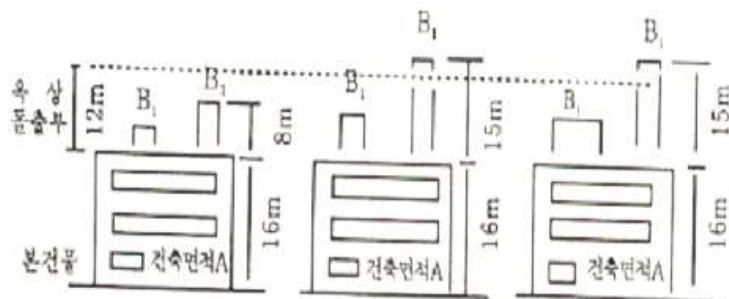
[그림 2-11] 옥상부분의 면적에 따른 건축물의 높이 산정
