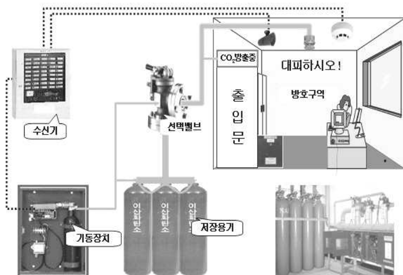
[그림 6-2] 이산화탄소소화설비 구성요소
