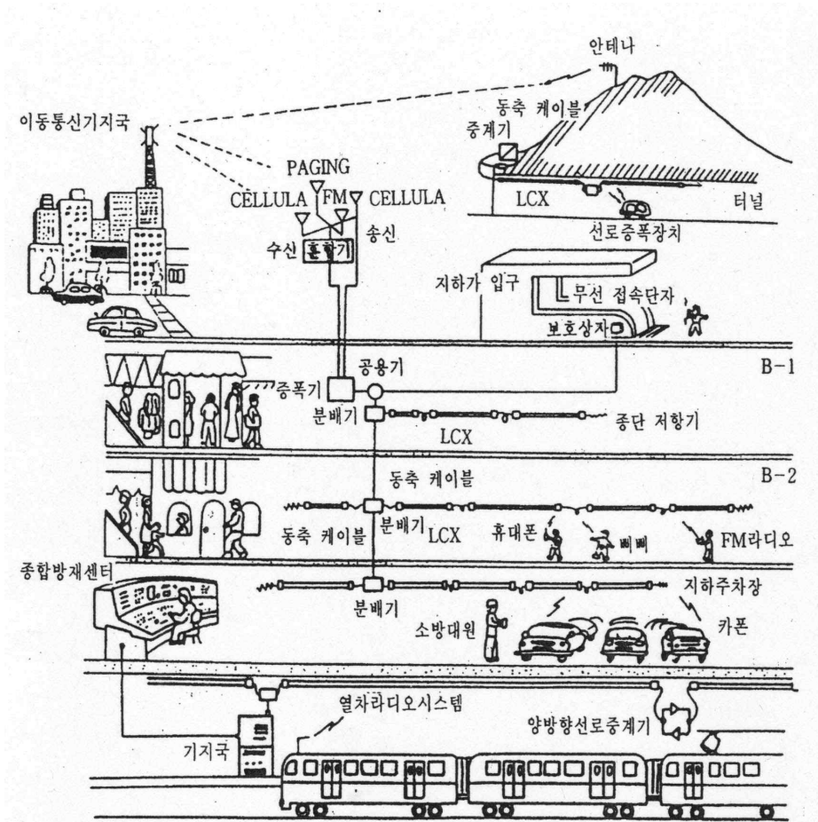
[그림 3-19] 무선통신보조설비의 사용
