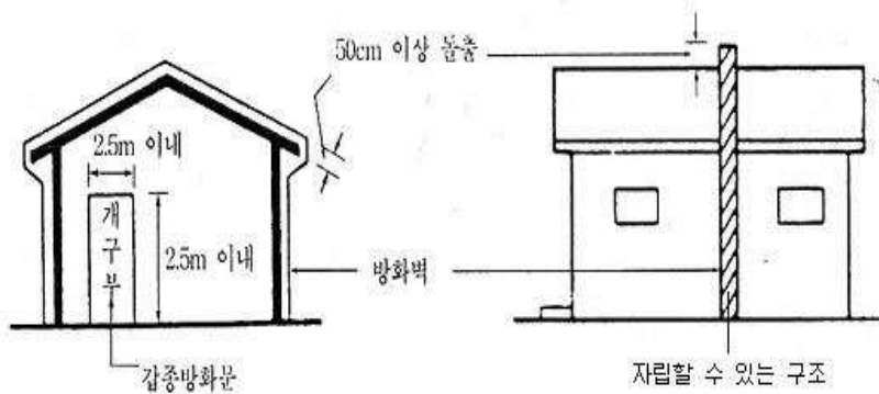
[그림 3-2] 방화벽 설치
