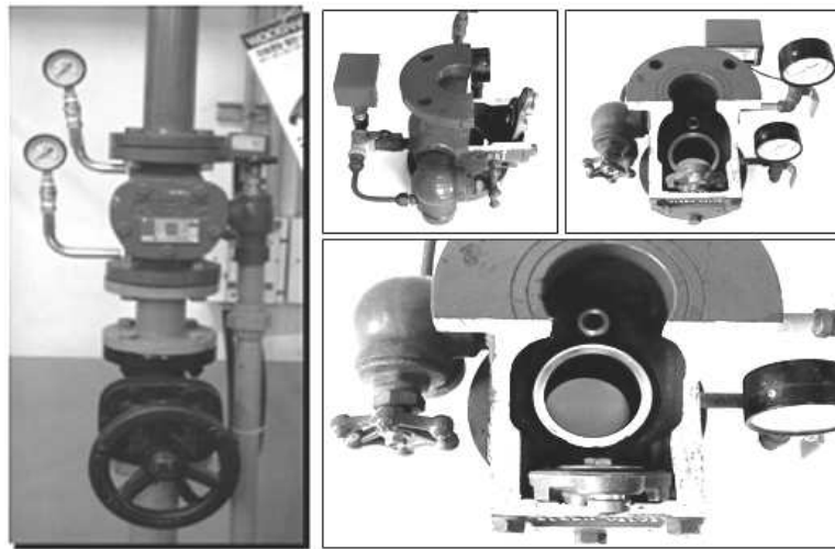
[그림 4-3] 습식밸브 구조
