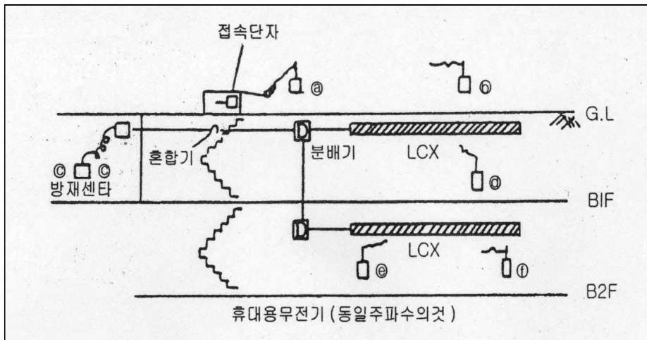
[그림 3-22] 무선통신보조설비의 사용
