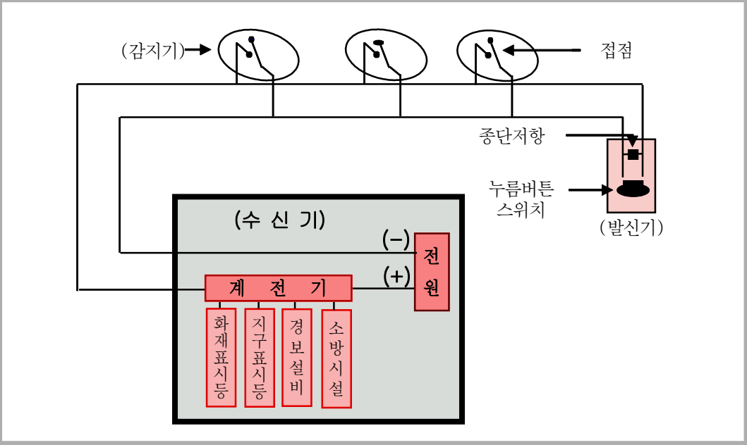
[그림 2-2] 자동화재탐지설비의 회로 간략도
