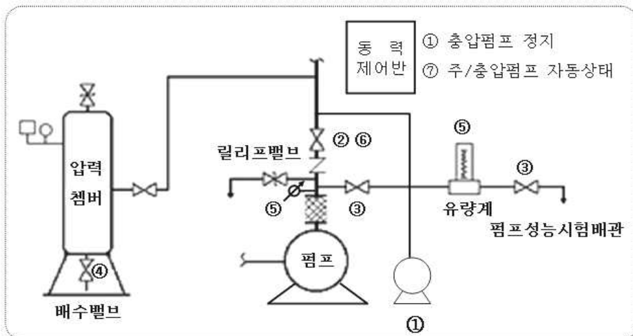
[그림 3-30] 펌프성능시험 방법
