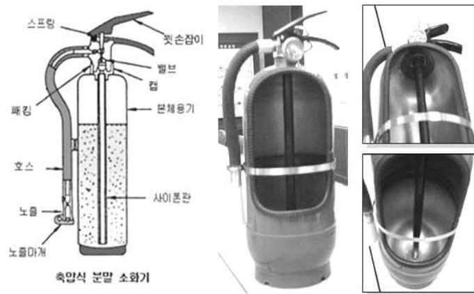
[그림 2-2] 축압식 분말소화기 구조
