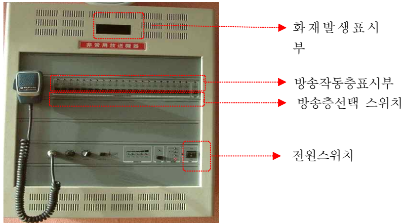
[그림 2-80] 비상방송설비의 스위치 및 표시등
