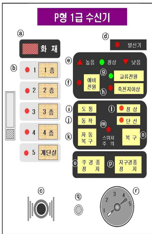
[그림 2-49] P형1급 수신기의 표시등 및 스위치
