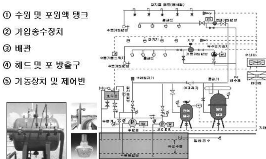
[그림 5-2] 포소화설비 구성요소
