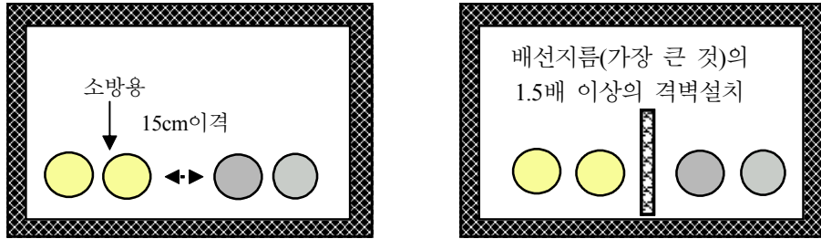
[그림 5-6] 내화배선 공사방법
