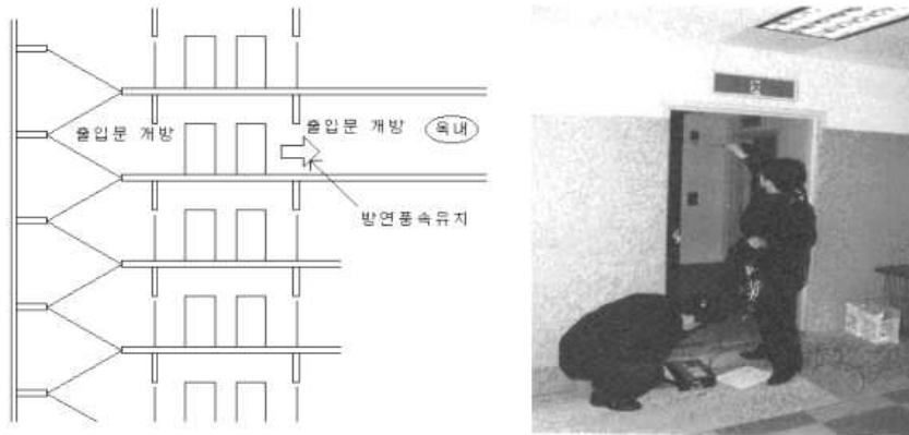
[그림 7-11] 방연풍속 측정
