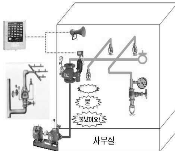
[그림 4-2] 스프링클러설비 구조 및 작동
