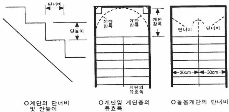
[그림 4-10] 계단의 구조
