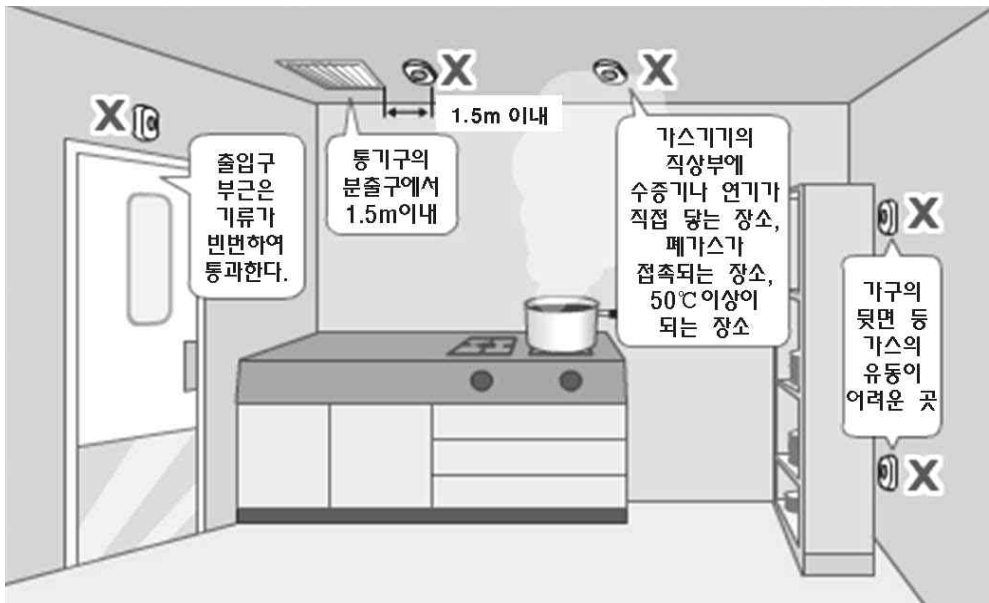
[그림 2-82] 가스누설경보기 검지기 설치장소
