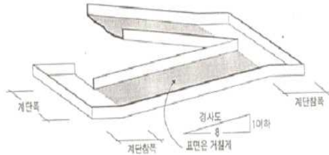
[그림 4-7] 경사로의 기준
