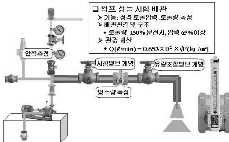
[그림 3-15] 펌프성능시험 배관
