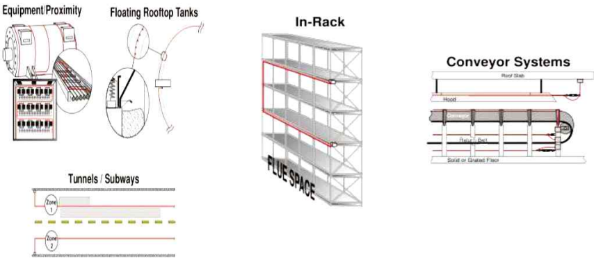
[그림 2-17] 정온식감지선형감지기 설치장소 예시
