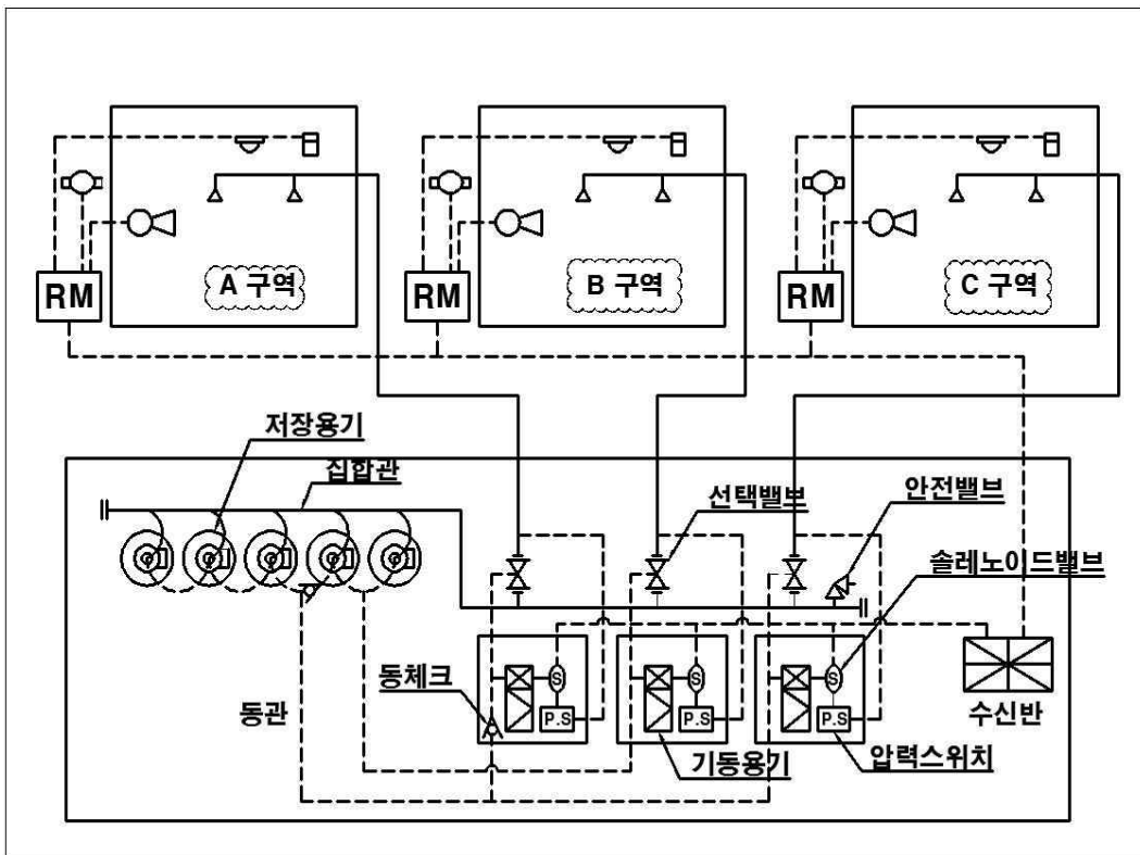
[그림 6-1] 이산화탄소설비 계통도
