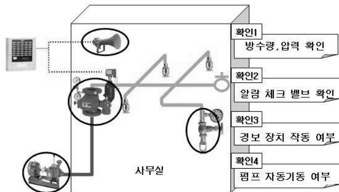
[그림 4-24] 습식스프링클러 점검사항
