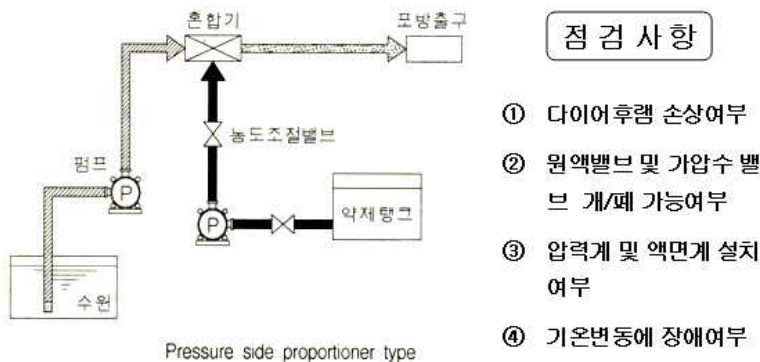
[그림 5-11] 프레저사이드프로포셔너 방식
