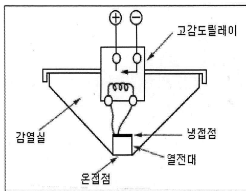
[그림 2-11] 열전대식감지기
