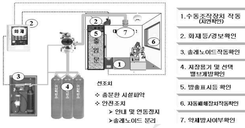
[그림 6-15] 기능점검 사항
