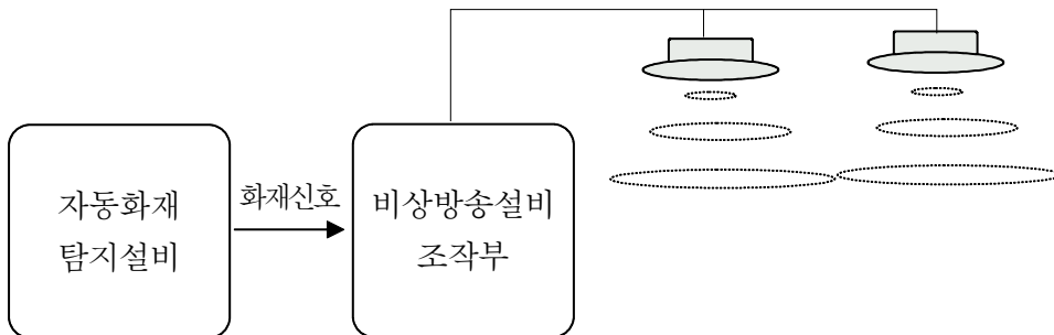
[그림 2-79] 비상방송설비의 작동흐름도
