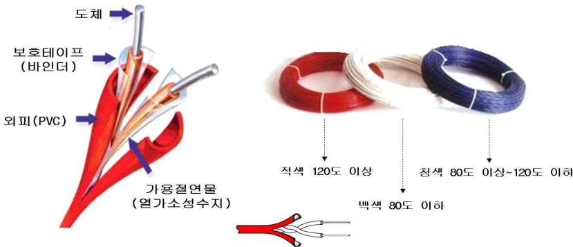
[그림 2-16] 정온식감지선형감지기의 형태 및 표시
