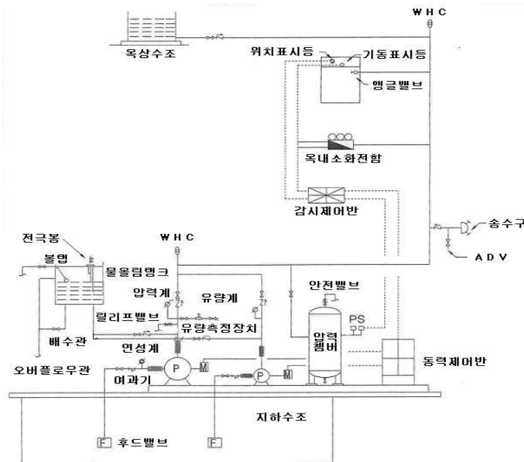
[그림 3-1] 옥내소화전 계통도 5)
