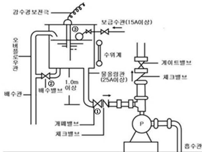
[그림 3-32] 자가발전설비 물올림 장치 점검
