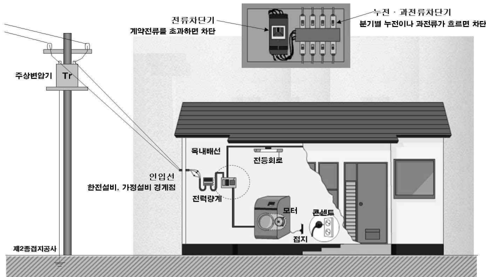
[그림 5-1] 일반주택의 옥내·외 배선
