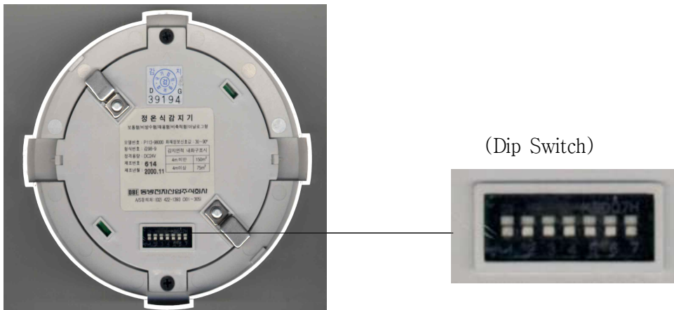
[그림 2-30] 주소형감지기의 주소지정
