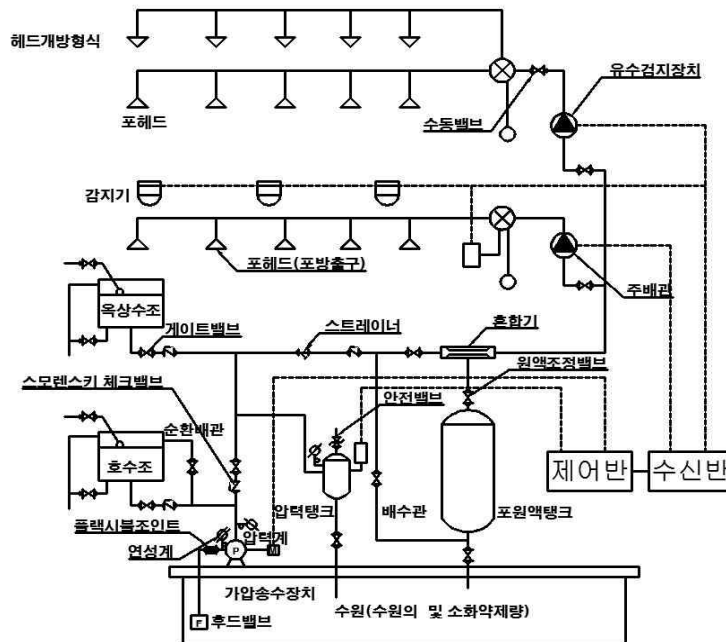
[그림 5-1] 포소화설비 계통도
