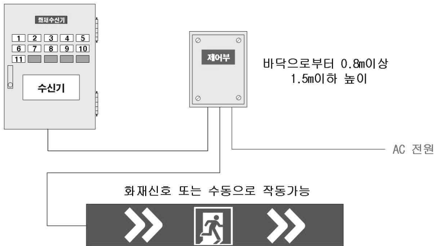
[그림 3-8] 광원점등방식 피난유도선 구성도
