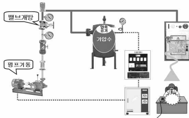
[그림 3-14] 압력챔버 구성과 기능
