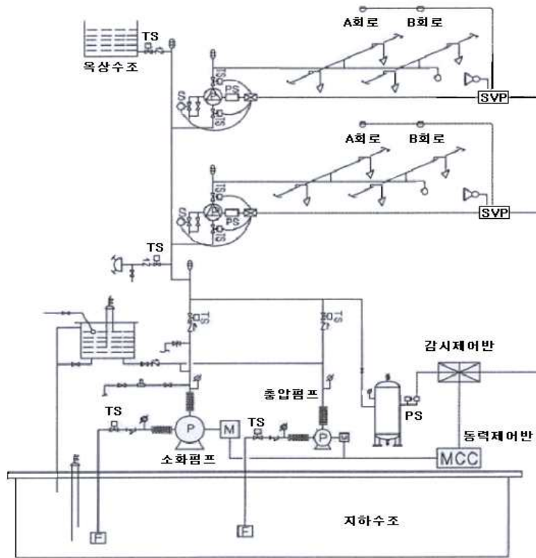
[그림 4-1] 준비작동식 스프링클러설비 계통도
