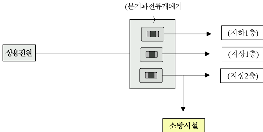
[그림 5-2] 소방시설 상용전원의 분기(×)
