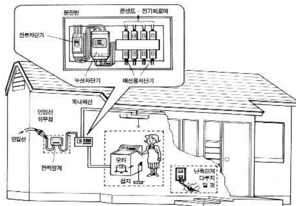
[그림 3-22] 상용전원 결선도
