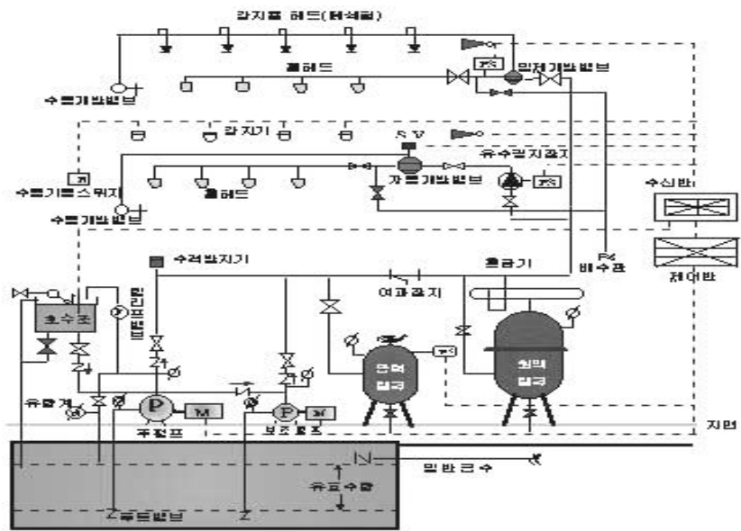
[그림 5-13] 홈헤드설비 방식
