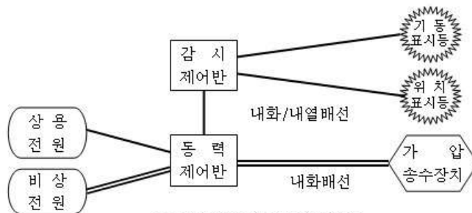
[옥내소화전/SP설비의 배선]
