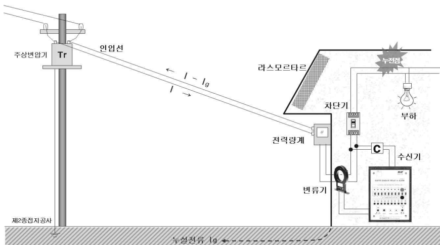
[그림 2-69] 누전경보기 설치구성도
