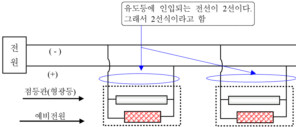
[그림 3-10] 2선식유도등의 배선
