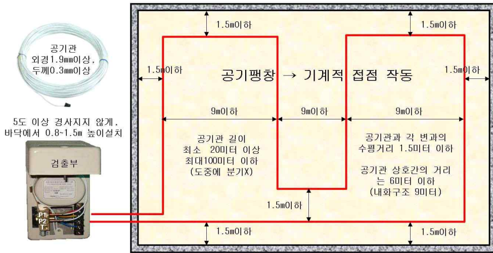
[그림 2-34] 공기관식 감지기의 설치기준
