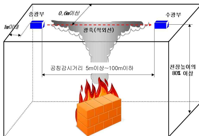
[그림 2-36] 광전식분리형감지기의 설치기준
