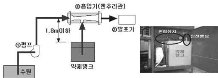
[그림 5-6] 라인프로포서너 방식
