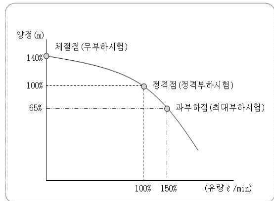
[소방펌프의 특성곡선]
