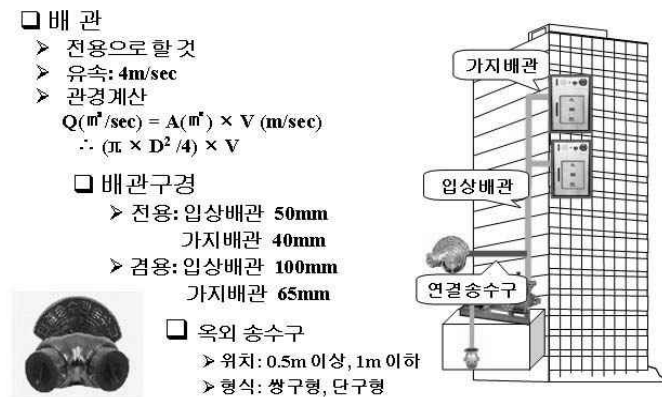
[그림 3-17] 배관 및 송수구
