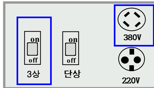
[그림 3-18] 비상콘센트함
