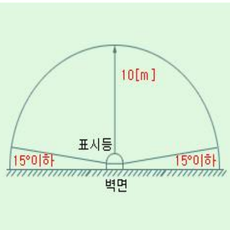
[그림 2-40] 표시등의 식별범위
