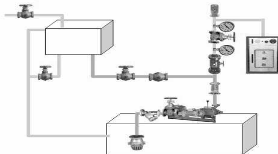
[그림 3-9] 물올림 장치 구조
