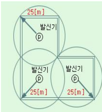
[그림 2-39] 발신기의 설치거리
