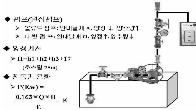
[그림 3-13] 펌프방식의 전동기 용량
