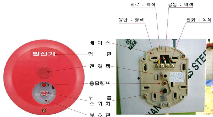
[그림 2-38] 발신기 구성
