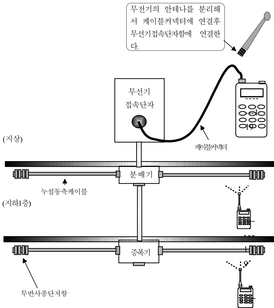
[그림 3-20] 무선통신보조설비의 구성
