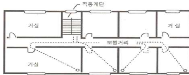
[그림 4-4] 직통계단까지 보행거리
