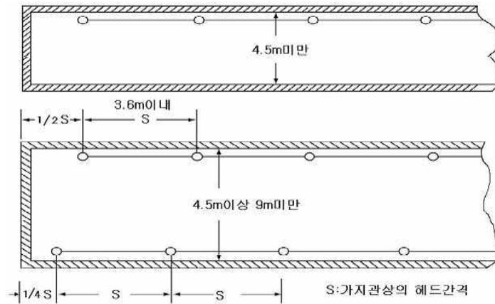
[그림 4-23] 측벽형 헤드설치
