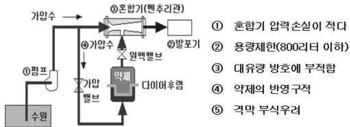
[그림 5-8] 격막이 있는 방식
