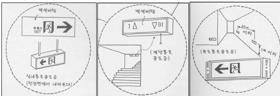
[그림 3-5] 통로유도등의 설치 기준
