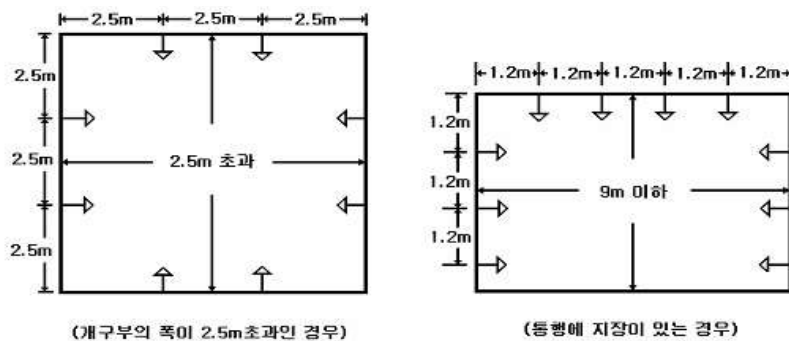
[그림 4-22] 연소할 개구부의 헤드설치
