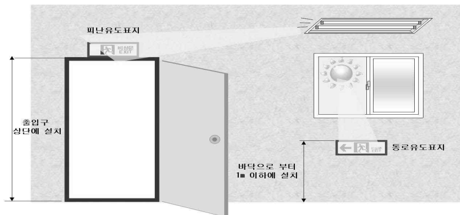
[그림 3-7] 유도표지 설치기준
