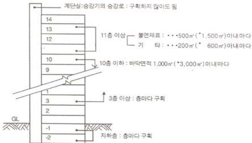
[그림 3-1] 방화구획 설치기준
