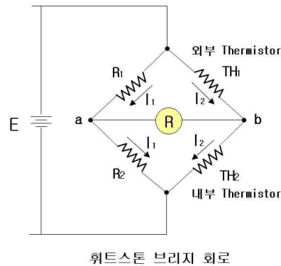
[그림 2-12] 열반도체식감지기
