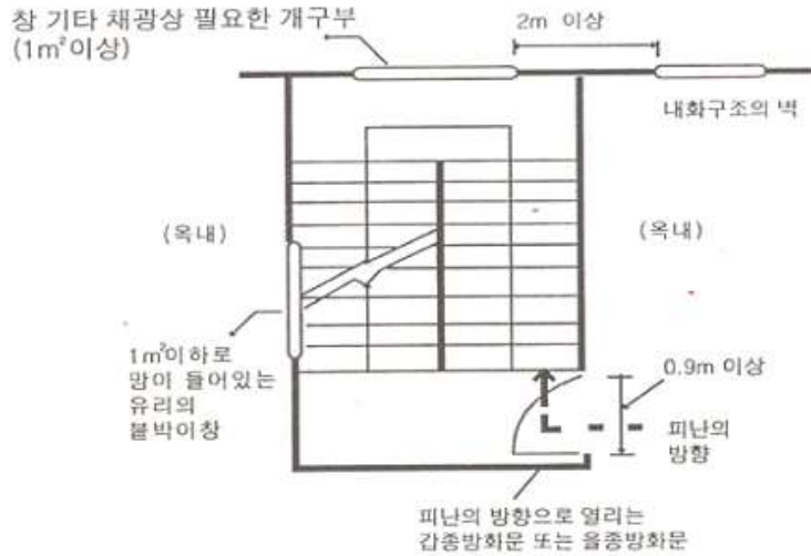
[그림 4-12] 옥내피난계단의 구조
