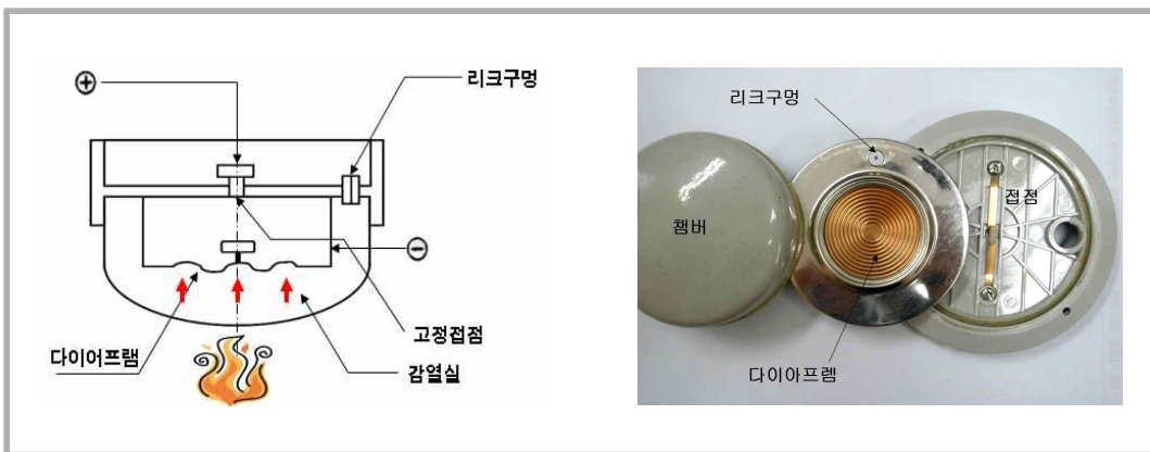
[그림 2-4] 차동식스포츠형 감지기 구조
