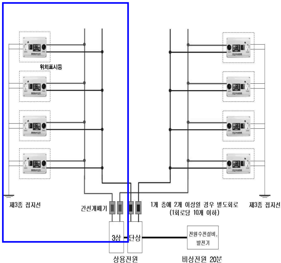
[그림 3-16] 비상콘센트설비의 배선도
