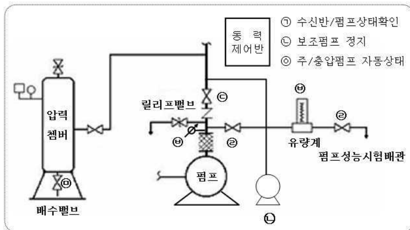
[그림 3-16] 펌프성능시험 방법
