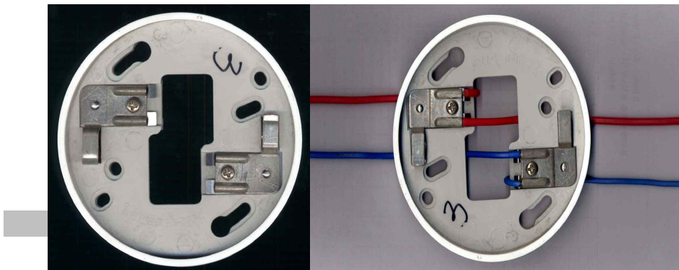
[그림 2-8] 감지기 베이스 및 배선방법
