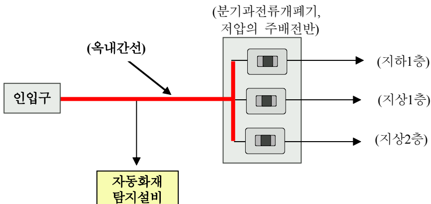
[그림 5-4] 자동화재탐지설비 상용전원의 분기
