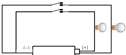
[그림 8] 공통선 배선
