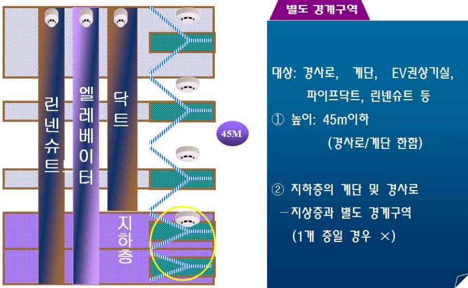
[그림 3] 수평적, 수직적 경계구역 예시
