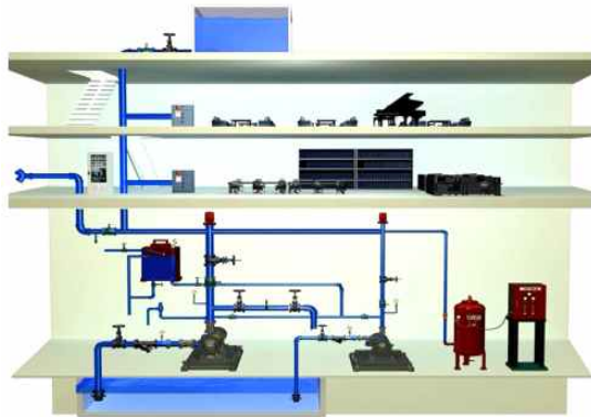
[건축물에 설치되는 펌프(지하수조)를 이용하는 급수방식 예]
