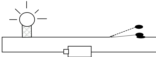
[그림4] 점점신호
