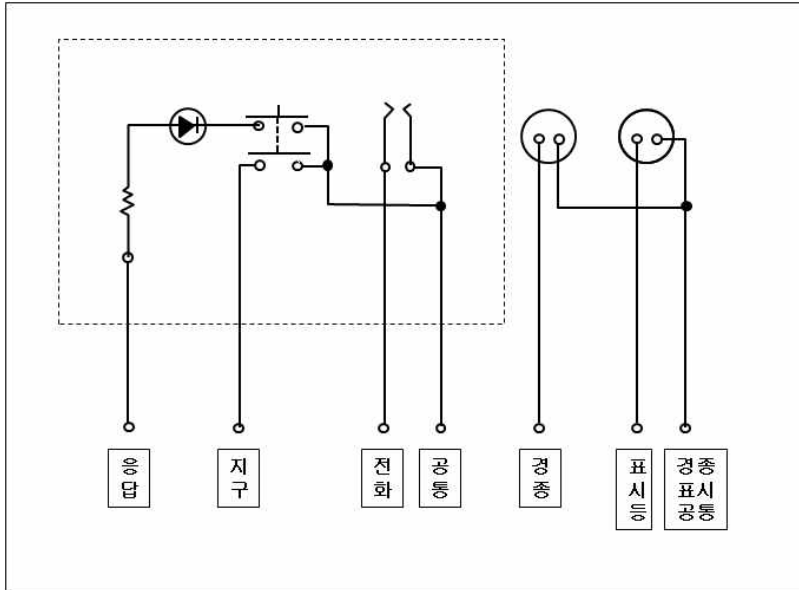
[그림 10] 경계구역 회로
